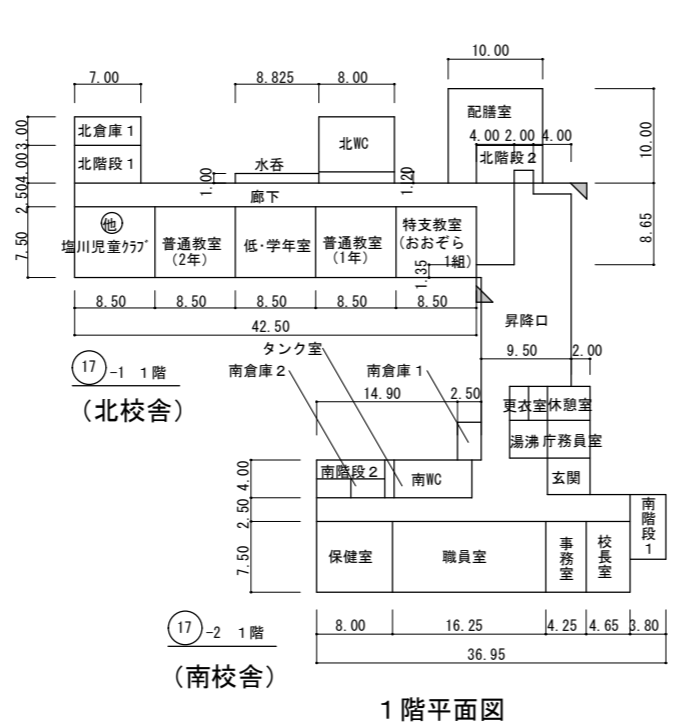
17-1 普通教室棟 平面図 S=1/800 (北校舎)
