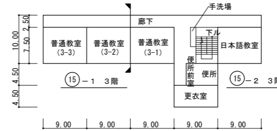
3階平面図
