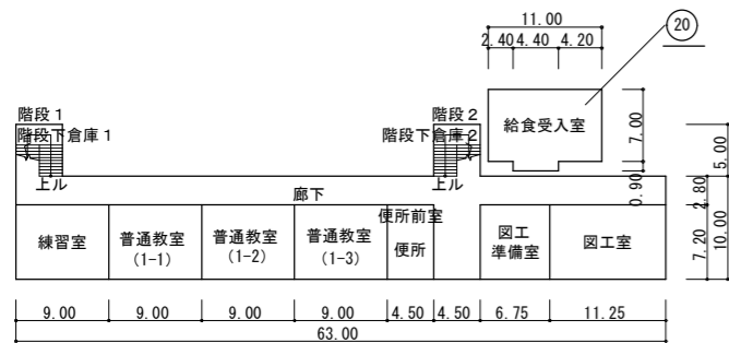
1階平面図
