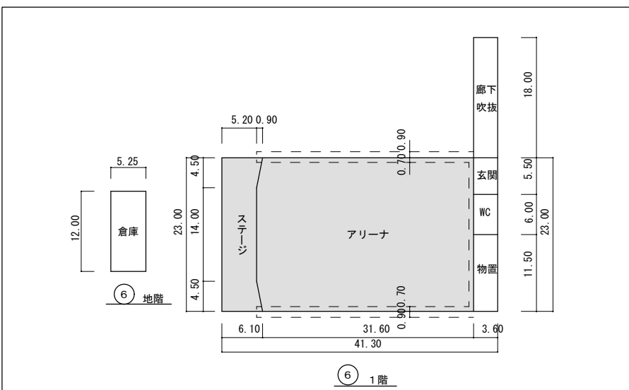
⑥ 屋内運動場 平面図 S=1/800
