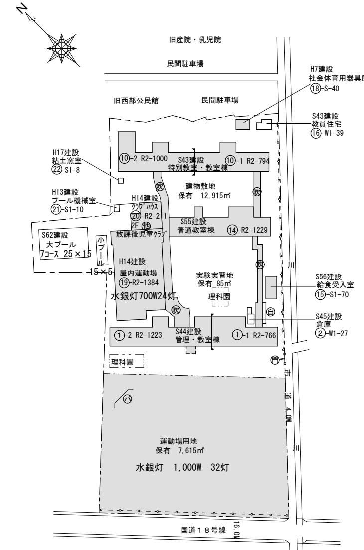
西小 配置図 S=1/2,000
