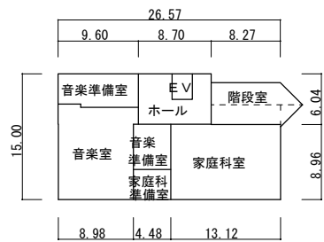
12-2 2階
