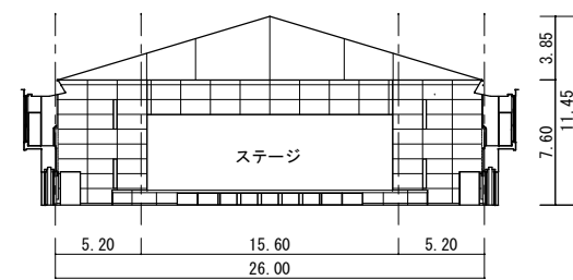
19 屋内運動場 展開図 S=1/500
