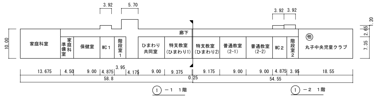
1階平面図
