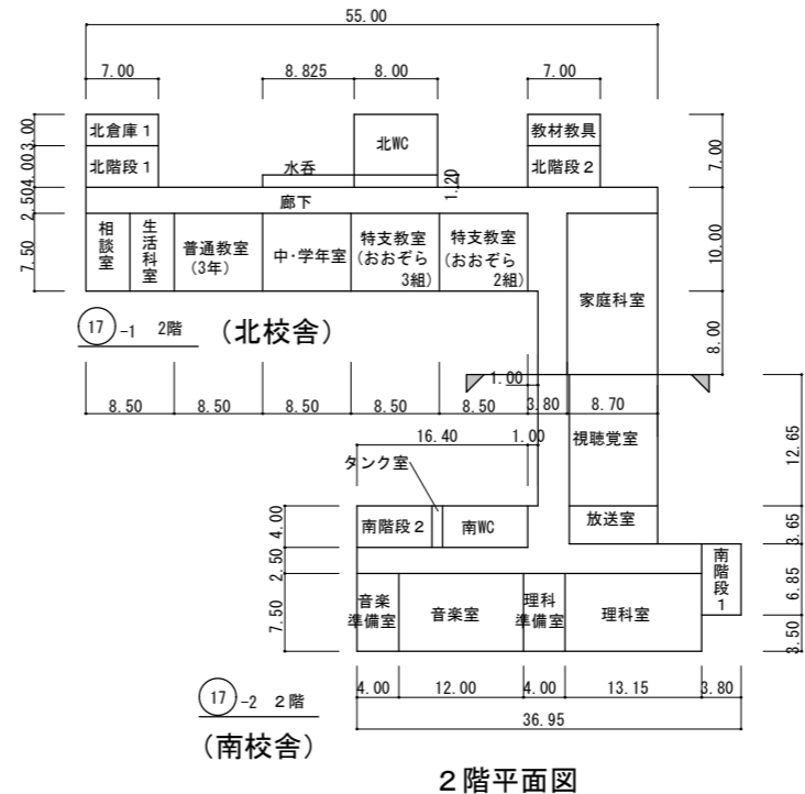
17-2 管理・特別教室棟 平面図 S=1/800 (南校舎)
