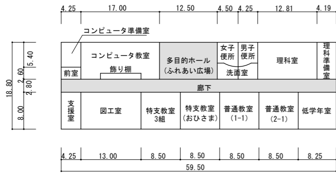
② 1階平面図
