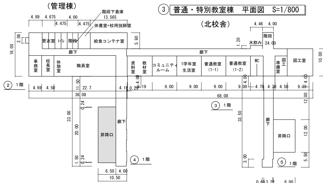
4 昇降口棟 平面図 S=1/800
