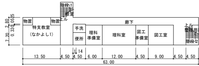
16-2 1階
