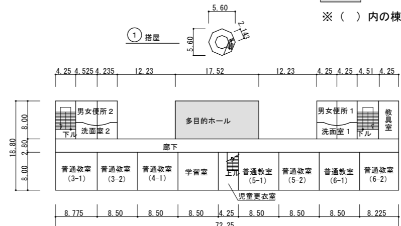
① 2階平面図
