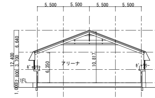
⑨ 屋内運動場 断面図 S=1/500
