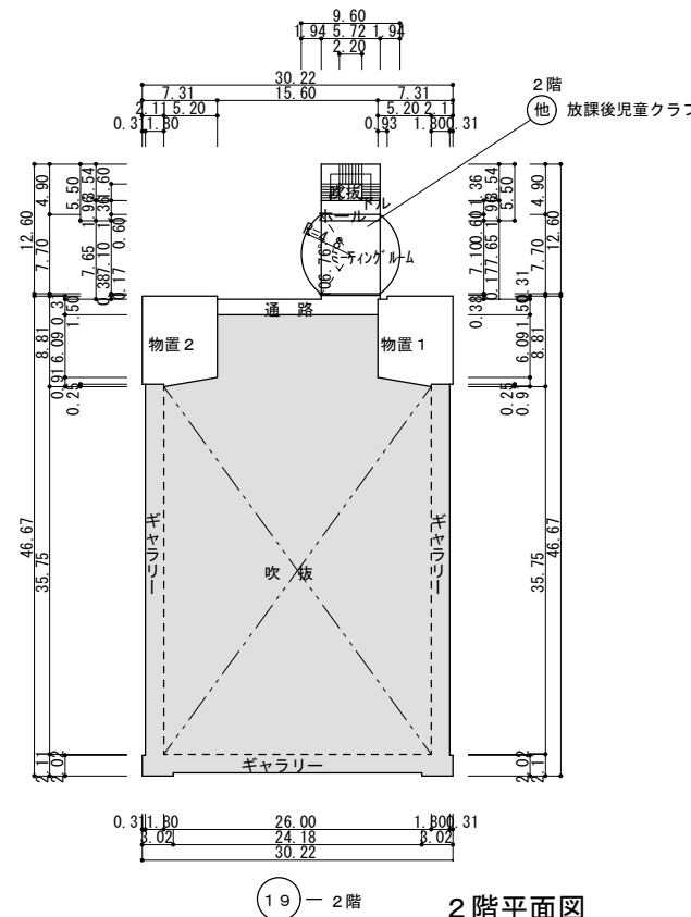
2階平面図
