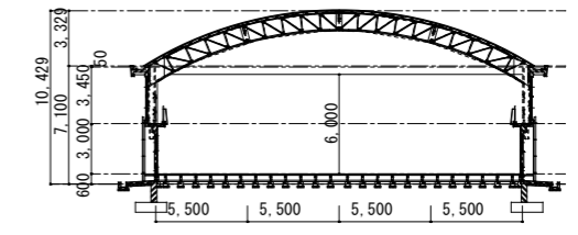
20 屋内運動場 矩計図 S=1/500
