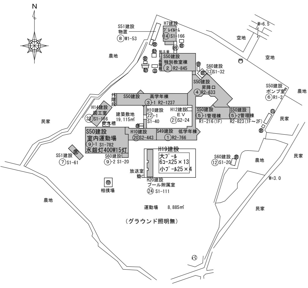
配置図 S=1/2,000
