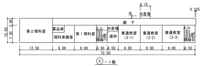
1階平面図
