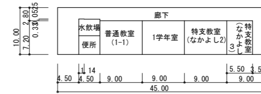
13 1階平面図
