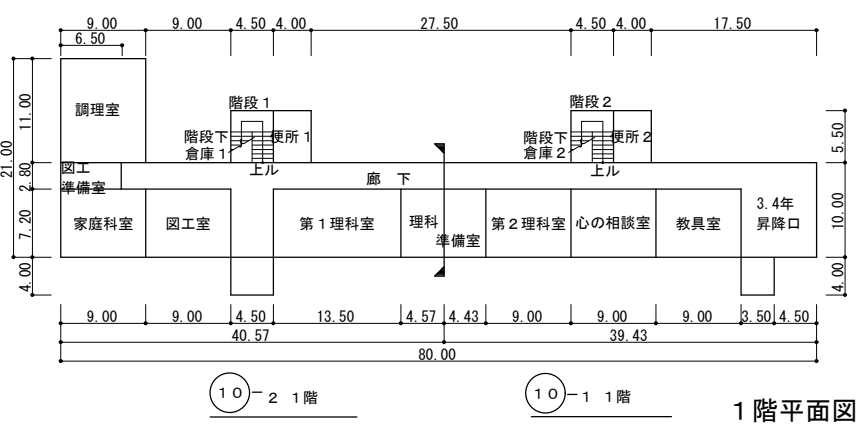
(10) 特別教室・教室棟 平面図 S=1/800 (北校舎)
