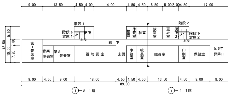
1階平面図
