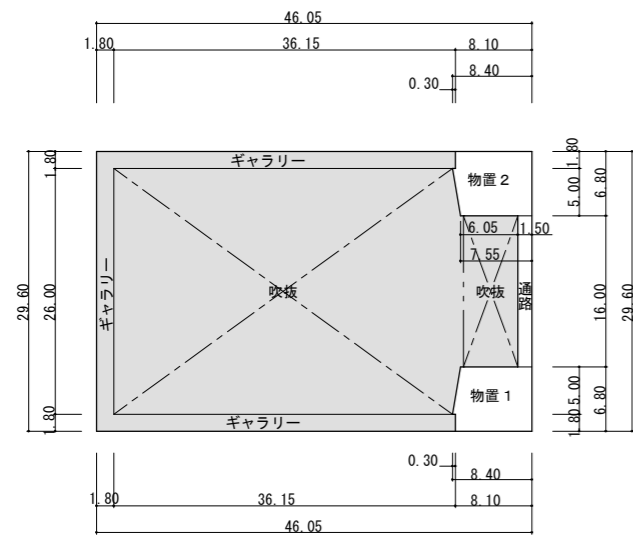
22 2階 2階平面図
