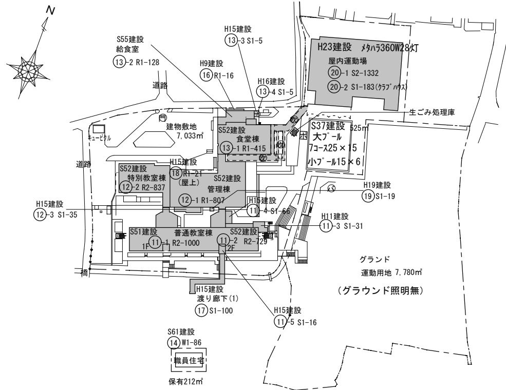
武石小 配置図 S=1/2,000
