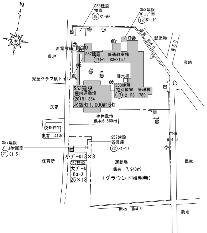
塩川小配置図 S=1/2,000
