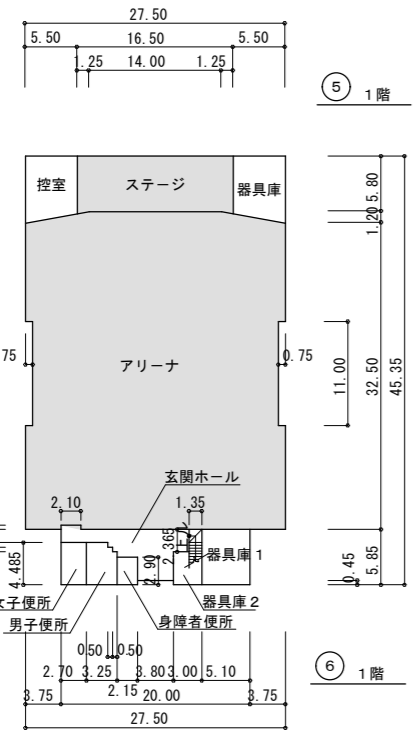
1階平面図
