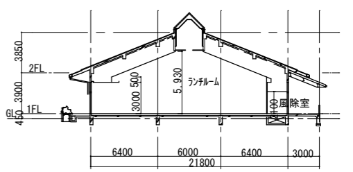
④ 学校食堂棟 断面図 S=1/500
