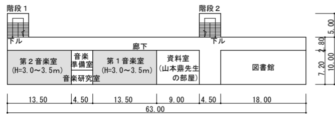
2階平面図
