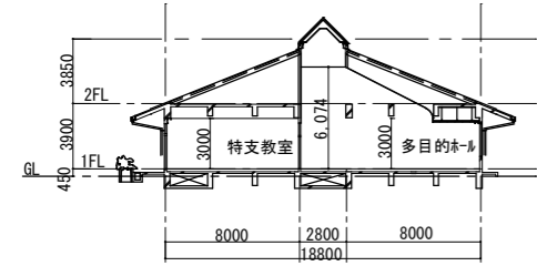
② 普通・特別教室棟 断面図 S=1/500
