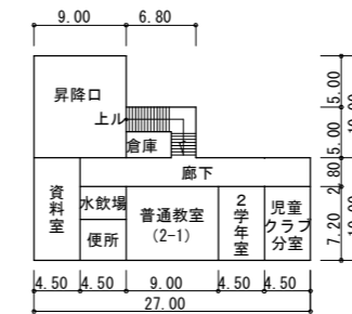
19 1階 1階平面図
