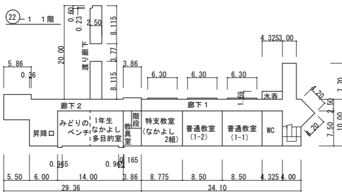
②0 1階 1階平面図
