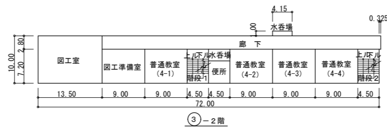
2階平面図
