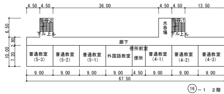
2階平面図
