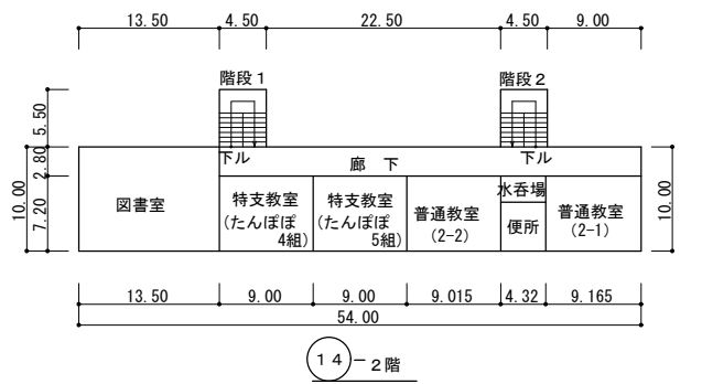
2階平面図
