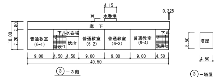
3階平面図
