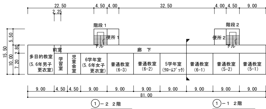
2階平面図
