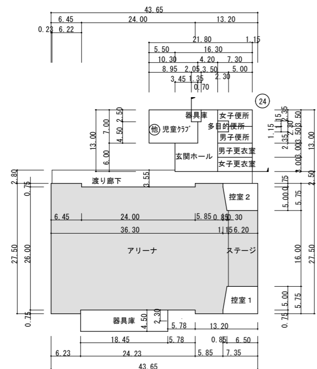
22 1階 1階平面図
