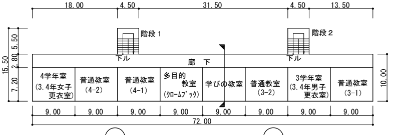
2階平面図
