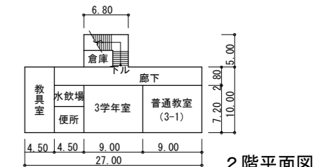
19 2階 2階平面図
