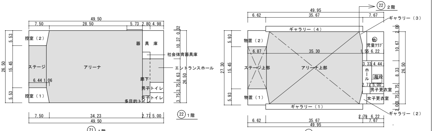
21 22 屋内運動場 平面図 S=1/800
