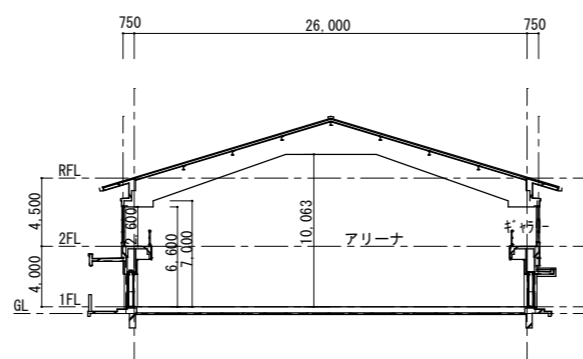
23 24 屋内運動場 断面図 S=1/500
