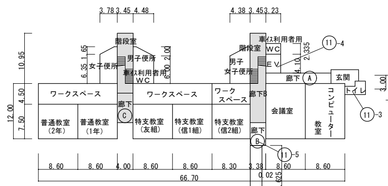
11-1 1階
