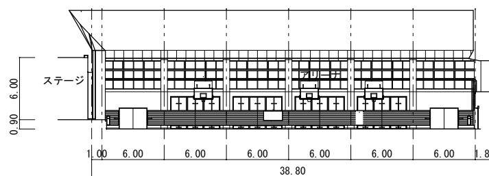
19 屋内運動場 展開図 S=1/500
