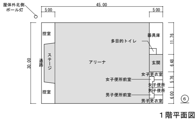
⑥ 屋内運動場 平面図 S=1/800
