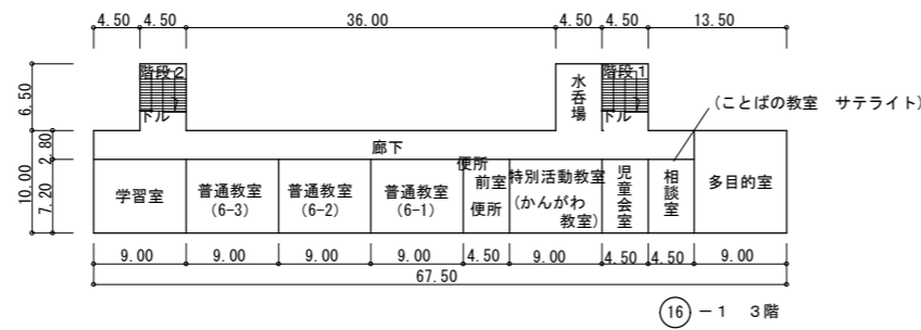
3階平面図
