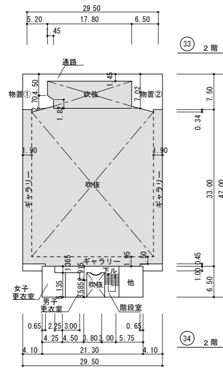
2階平面図
