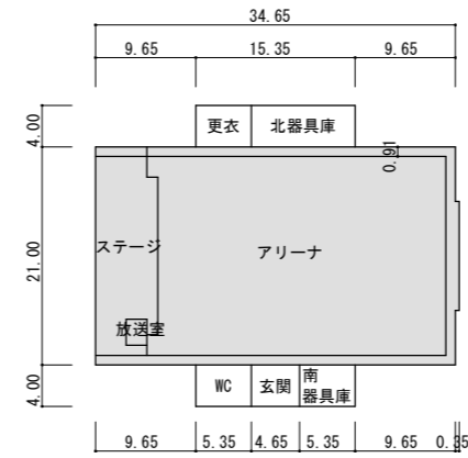
20 1階平面図
