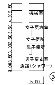
②4 プール附属室 平面図 S=1/800
