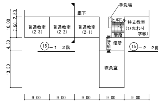
2階平面図
