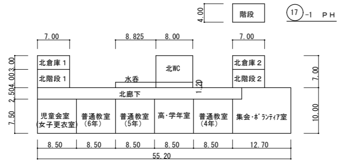
17-1 3階
