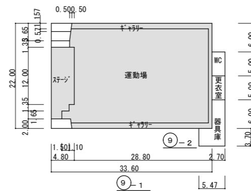
⑨ 屋内運動場 平面図 S=1/800
