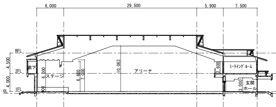
23 24 屋内運動場 断面図 S=1/500
