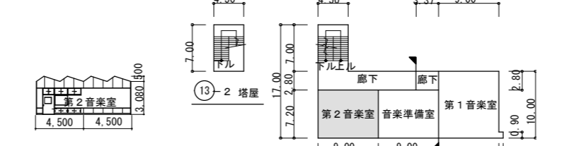
音楽室 展開図 S=1/500
