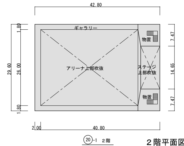
20 屋内運動場 平面図 S=1/800
