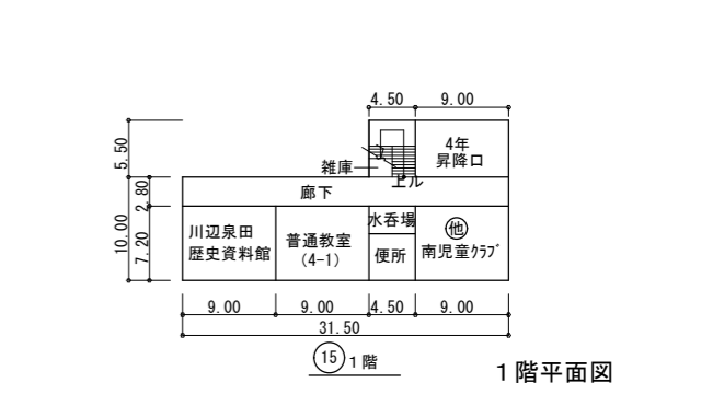
15 普通教室棟 平面図 S=1/800
