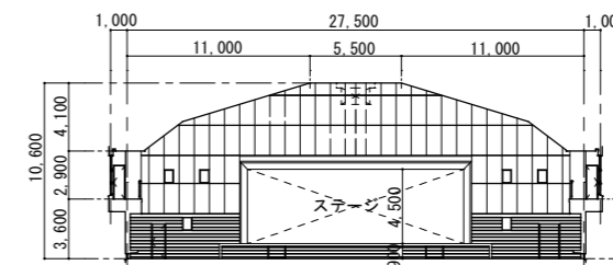
33 34 屋内運動場 展開図 S=1/500
