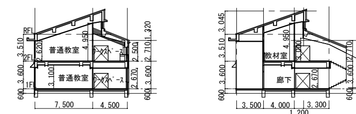
11 普通教室棟 断面図 S=1/500
