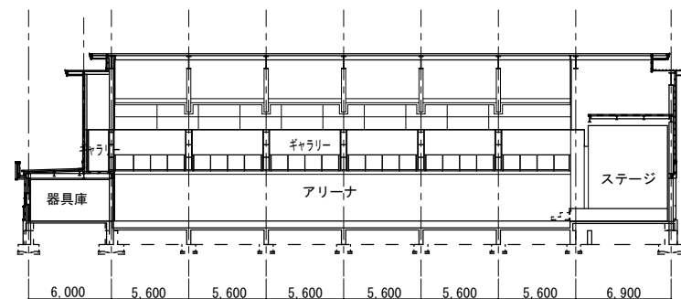
20 屋内運動場 断面図 S=1/500
