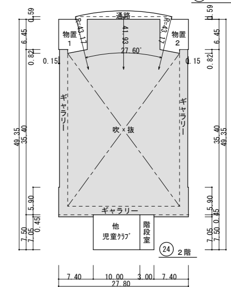
2階平面図
