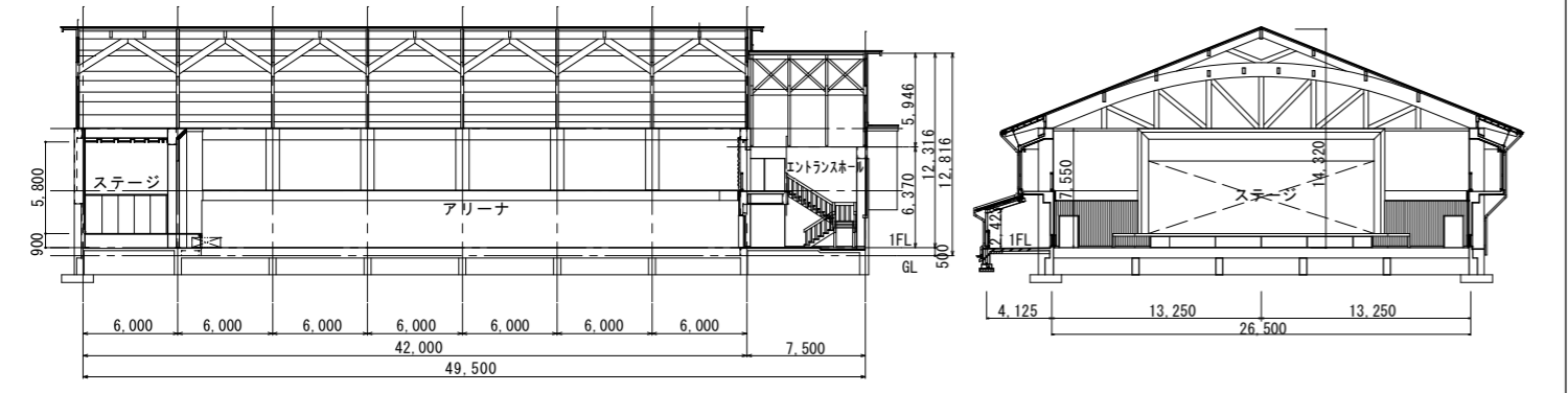
21 22 屋内運動場 展開図 S=1/500
