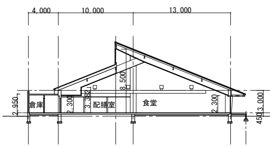
13 16 食堂棟 断面図 S=1/500
