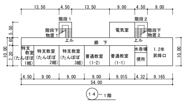
1階平面図
