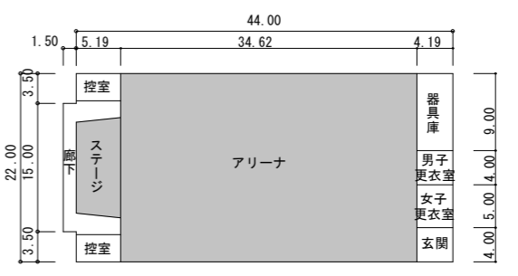
20 屋内運動場 平面図 S=1/800
