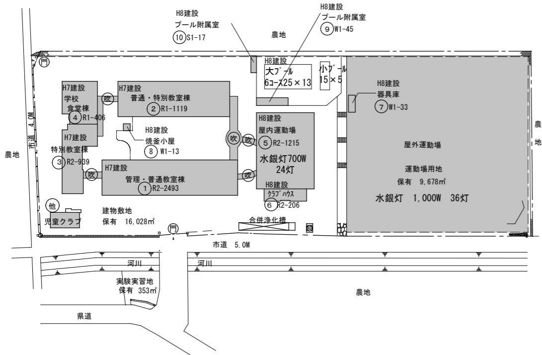
配置図 S=1/2,000
