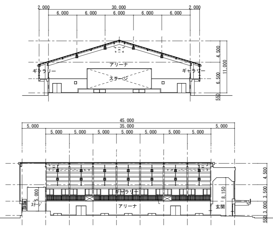
⑥ 屋内運動場 展開図 S=1/500
