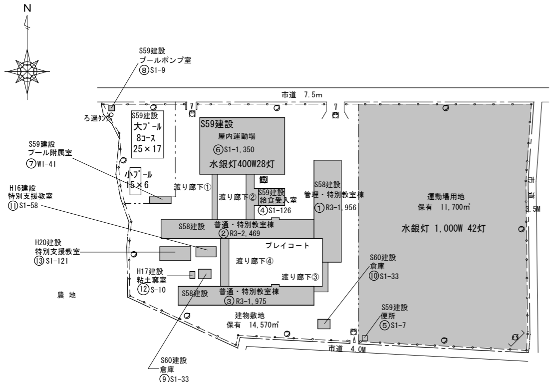
配置図 S=1/2,000
