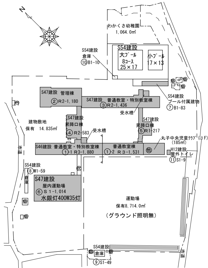
配置図 S=1/2,000
