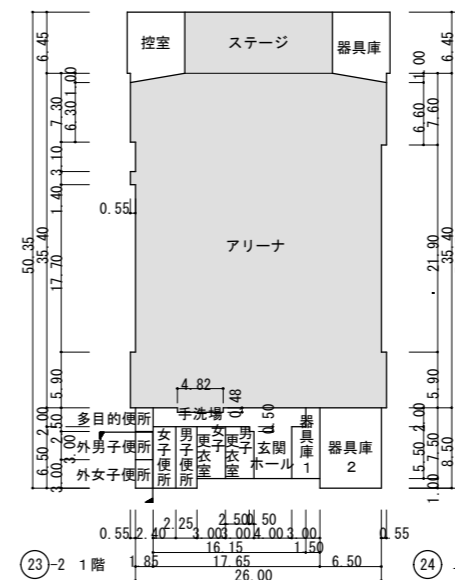
1階平面図
