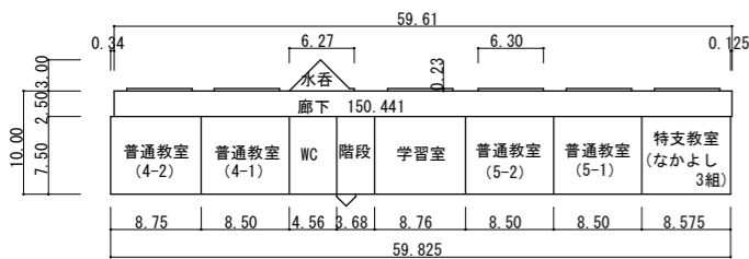
③-1 2階 2階平面図
