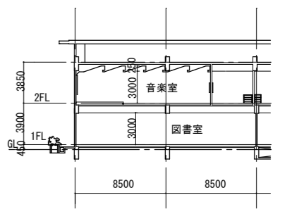
③ 特別教室棟 断面図 S=1/500
