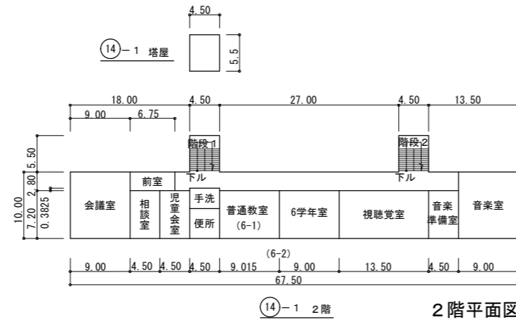
14 管理棟 平面図 S=1/800
