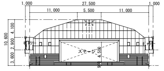
5 6 屋内運動場 展開図 S=1/500
