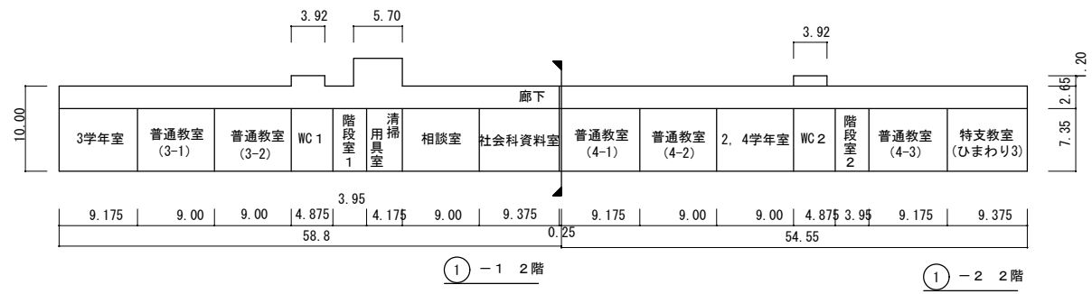
2階平面図
