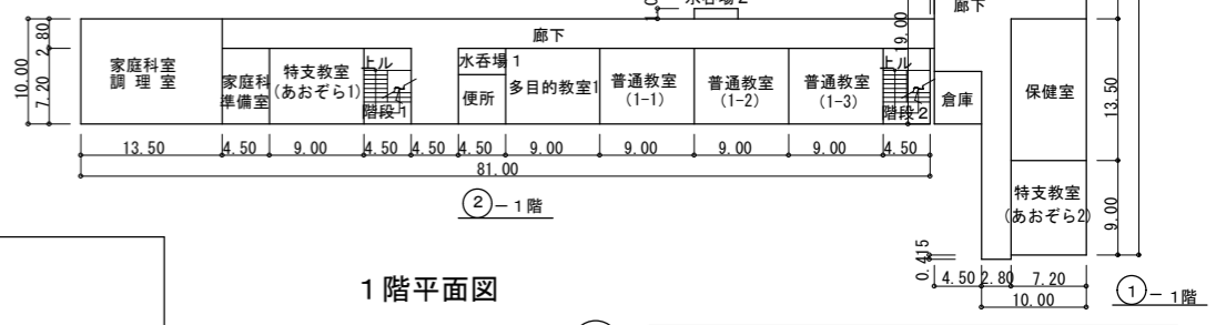
① 管理・特別教室棟 平面図 S=1/800 (東校舎)
