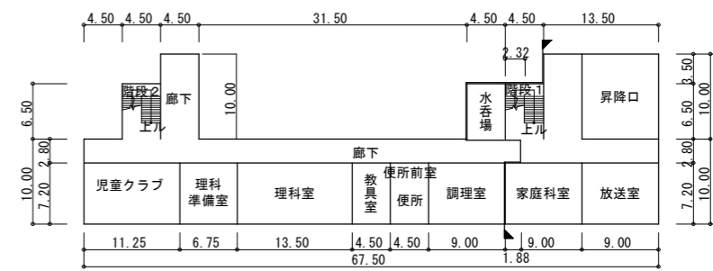
1階平面図
