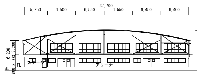
⑥ 屋内運動場 展開図 S=1/500
