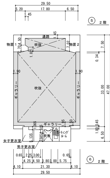
2階平面図
