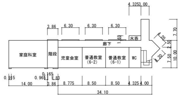
②0 2階 2階平面図
