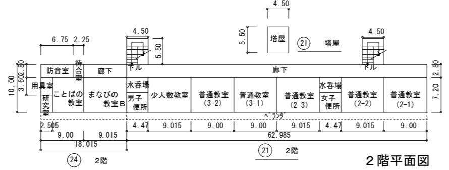
21 24 普通教室棟 平面図 S=1/800 (西校舎)
