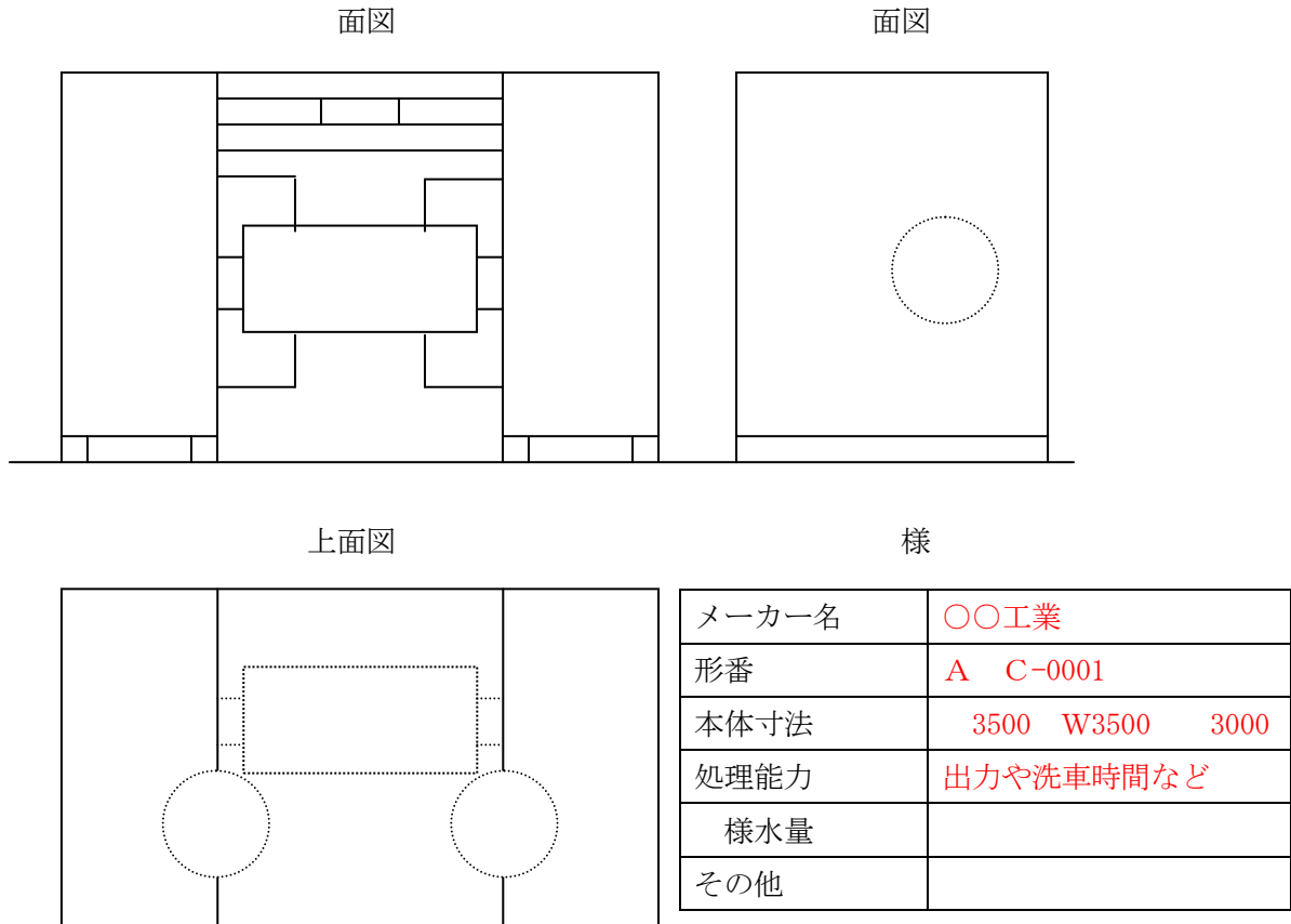
図一4 特定施設の構造図
