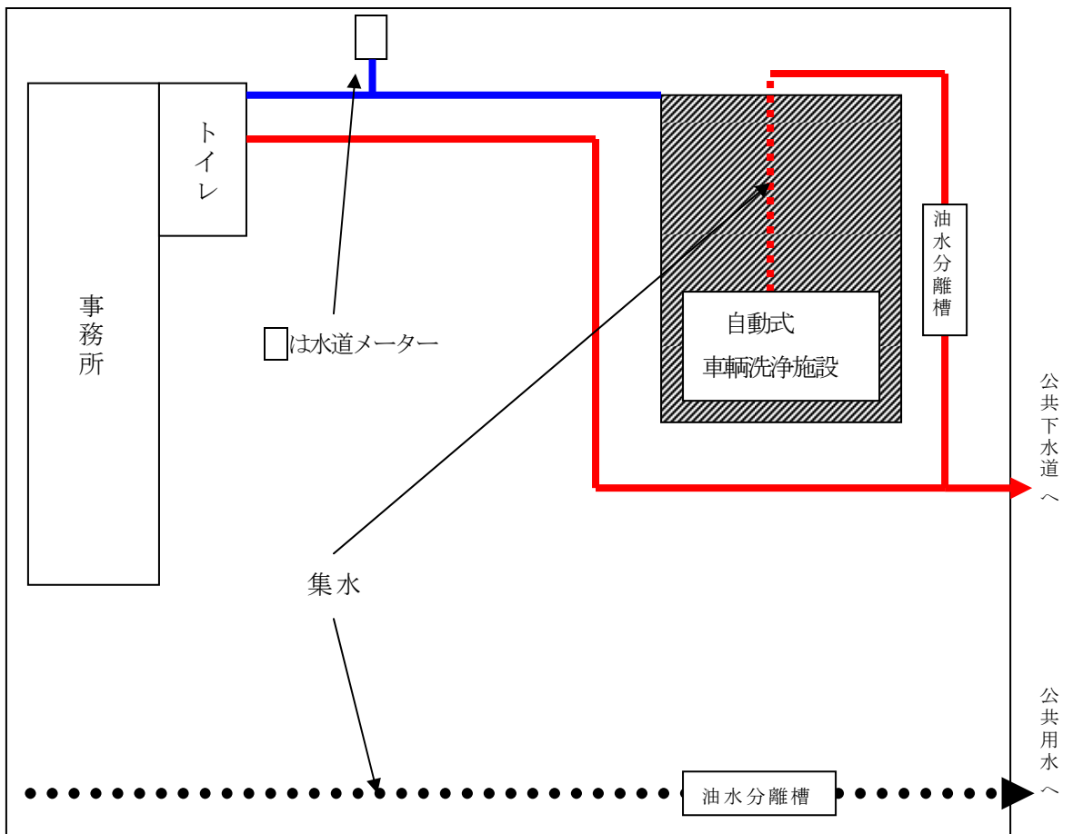
図一 3 特定施設等主要機器の配置図
