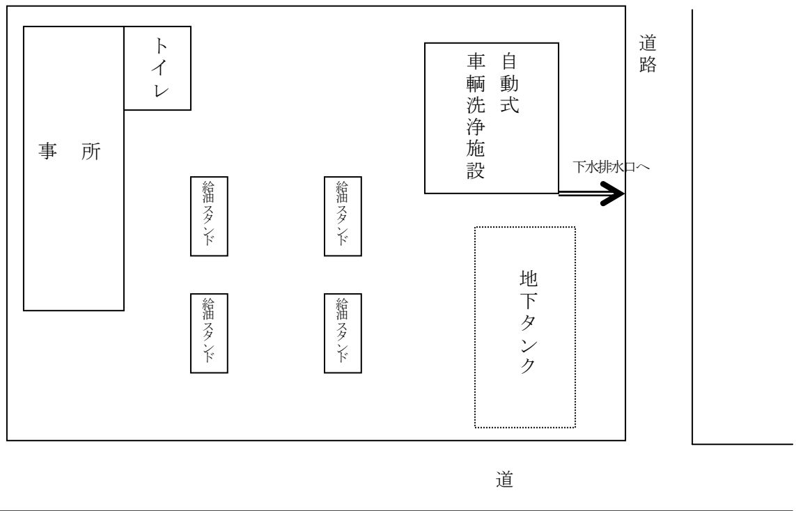
図一 3 特定施設等主要機器の配置図
