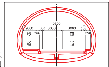
丸子小牧線バイパスのトンネルの断面図
