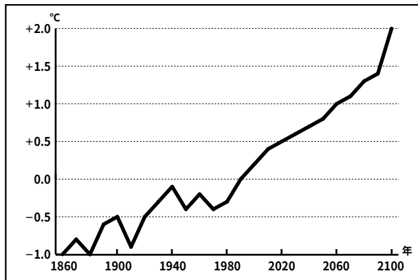
地球の平均気温の変化と予測
