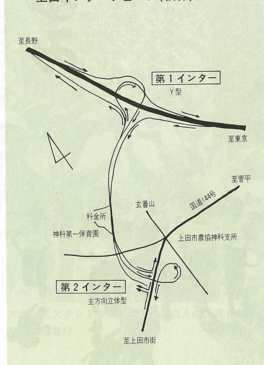
上田インターチェンジ(仮称)計画図
