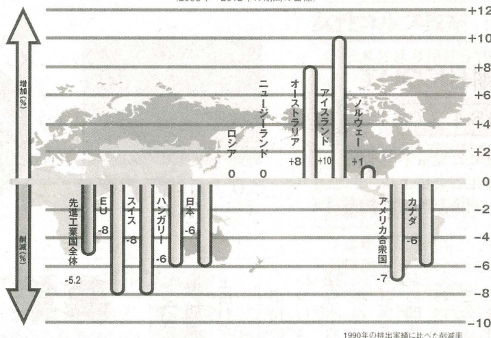
京都議定書で決められた主要国の温室効果ガス排出削減目標 (2008年～2012年の期間の目標)
