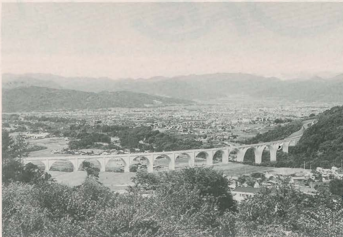
◀上信越自動車道 神川橋の予想写真。 神川を横過するこ の橋は鉄筋コンク リート連続アーチ 橋で、広視界性の 地形に調和した景 観を醸し出してい ます。この型式の 橋では日本で最長 (714.5m)となりま す。
