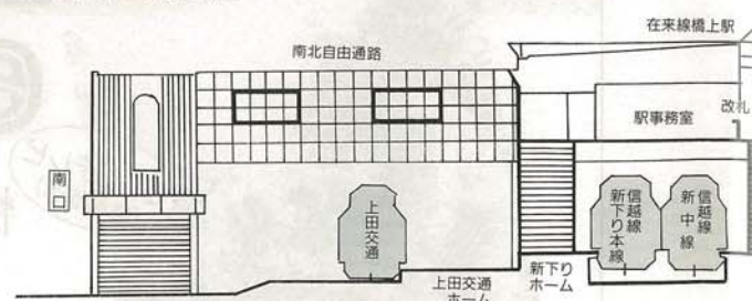
上田駅計画断面図
