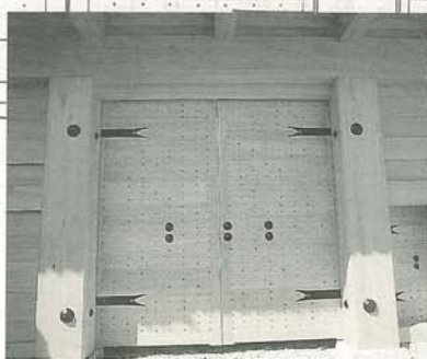
←観音開きの大戸は、1枚が高さ約4メートル、幅約2メートル、重さ約650キロ
