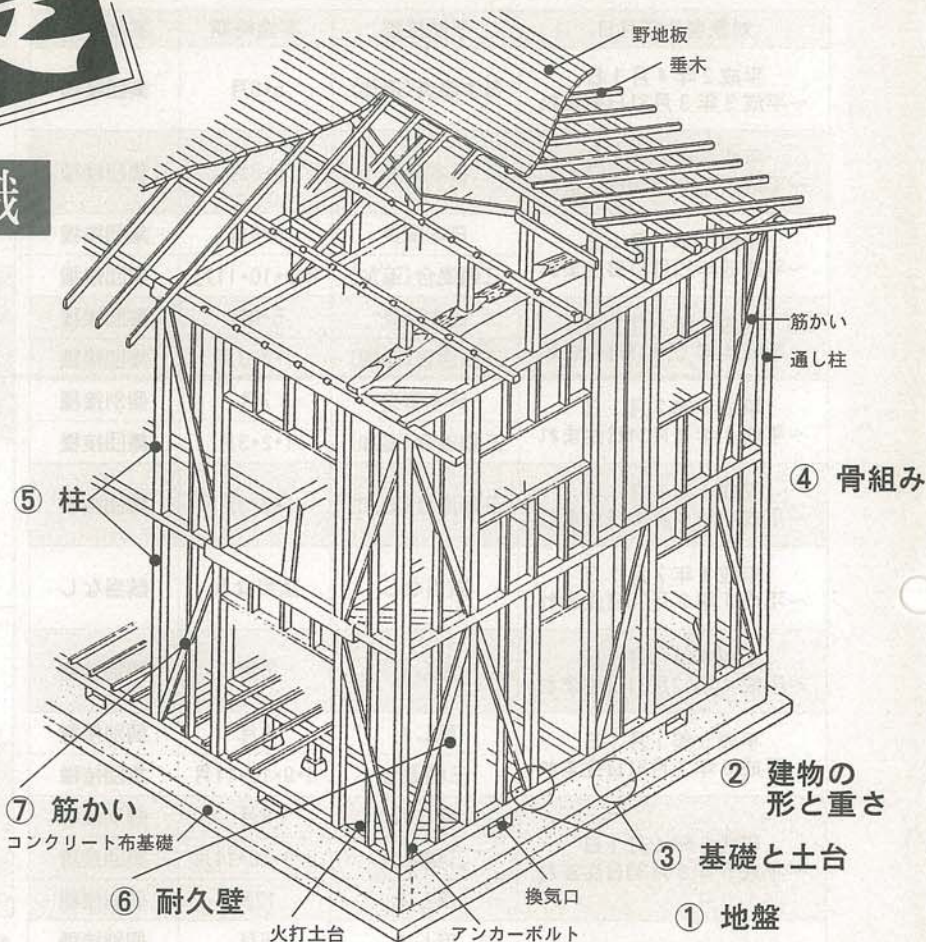
木造住宅の軸組図の例
