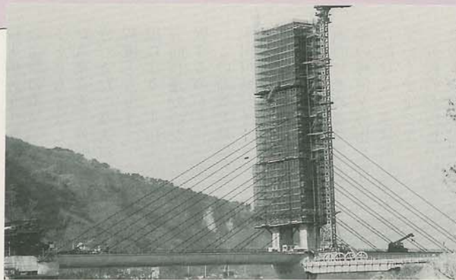
建設が進む、北陸新幹線第2千曲川橋りょう
