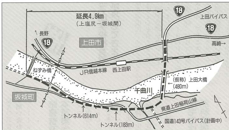
(仮称)上田大橋を上塩尻・下之条間に建設予定
