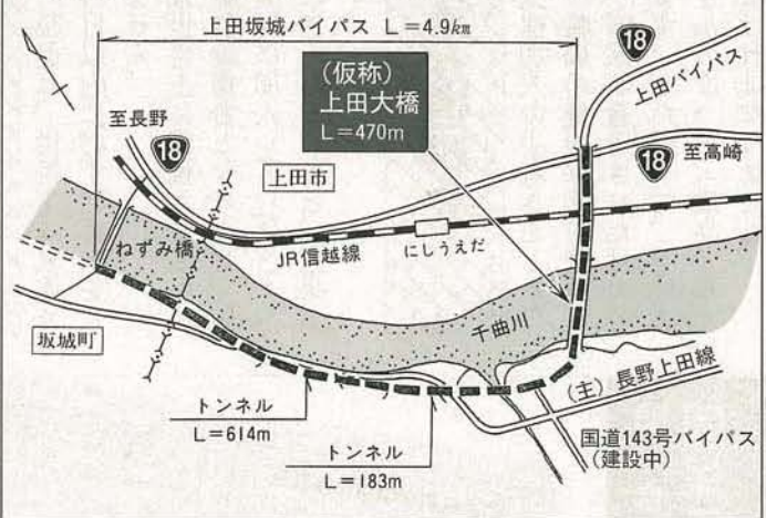
■ (仮称) 上田大橋および上田坂城バイパス計画図
