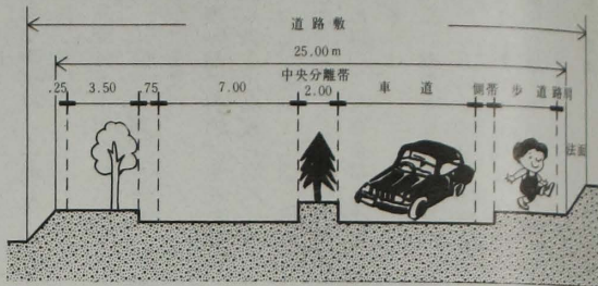
国道上田バイパス横断面図
