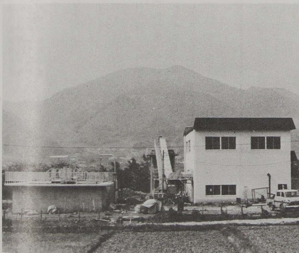
染屋浄水場に建設している汚泥処理施設は今秋の完成を目指して工事が進められています。写真は、汚水濃縮そう(左)と機械室(右)が姿を現わした工事現場。
