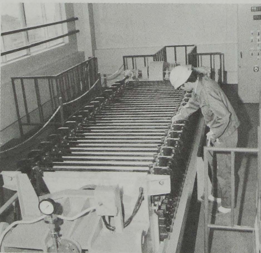
染屋浄水場の泥水処理に活躍する全自動脱水機
