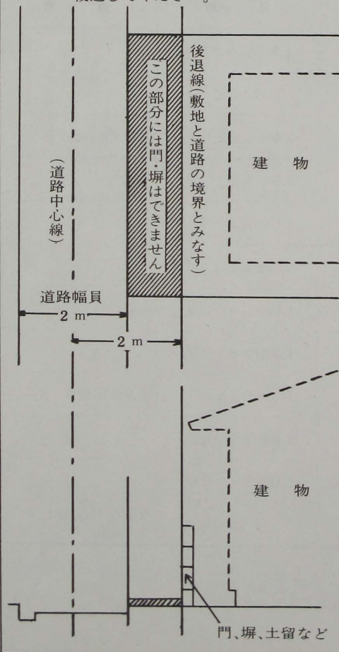
図① 道路幅員が1.8m以上4.0m未満の場合には、道路の中心線から2.0m後退してください。
