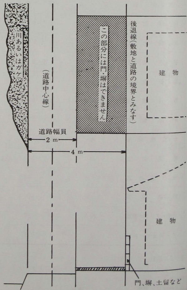
図② 道路の反対側に川やガケなどがある場合にはその境界線から4.0m後退してください。
