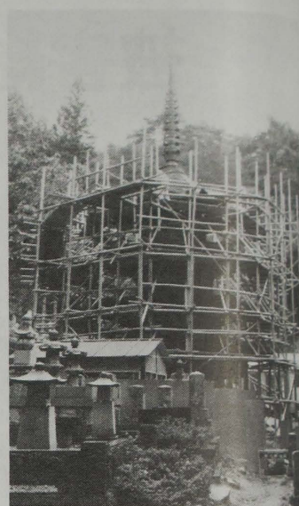
12月完成を目指して進められている 安楽寺八角三重塔の改修工事
