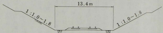
切取 (バラスト軌道の場合)
