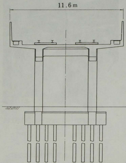
高架橋
