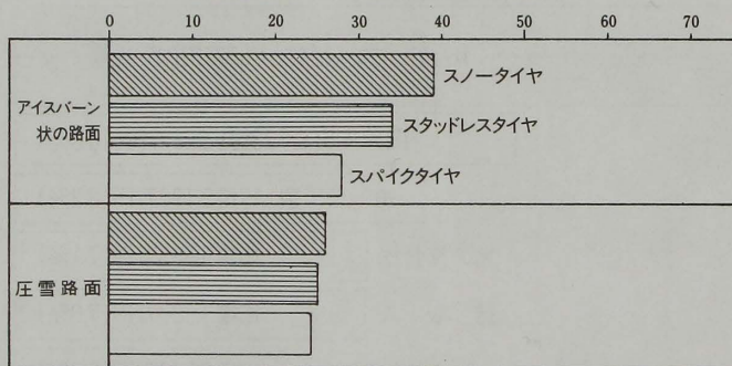
時速50kmでの制動停止距離(m)
