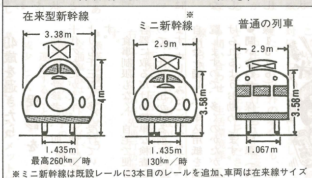
新幹線建設の各手法（図①）
