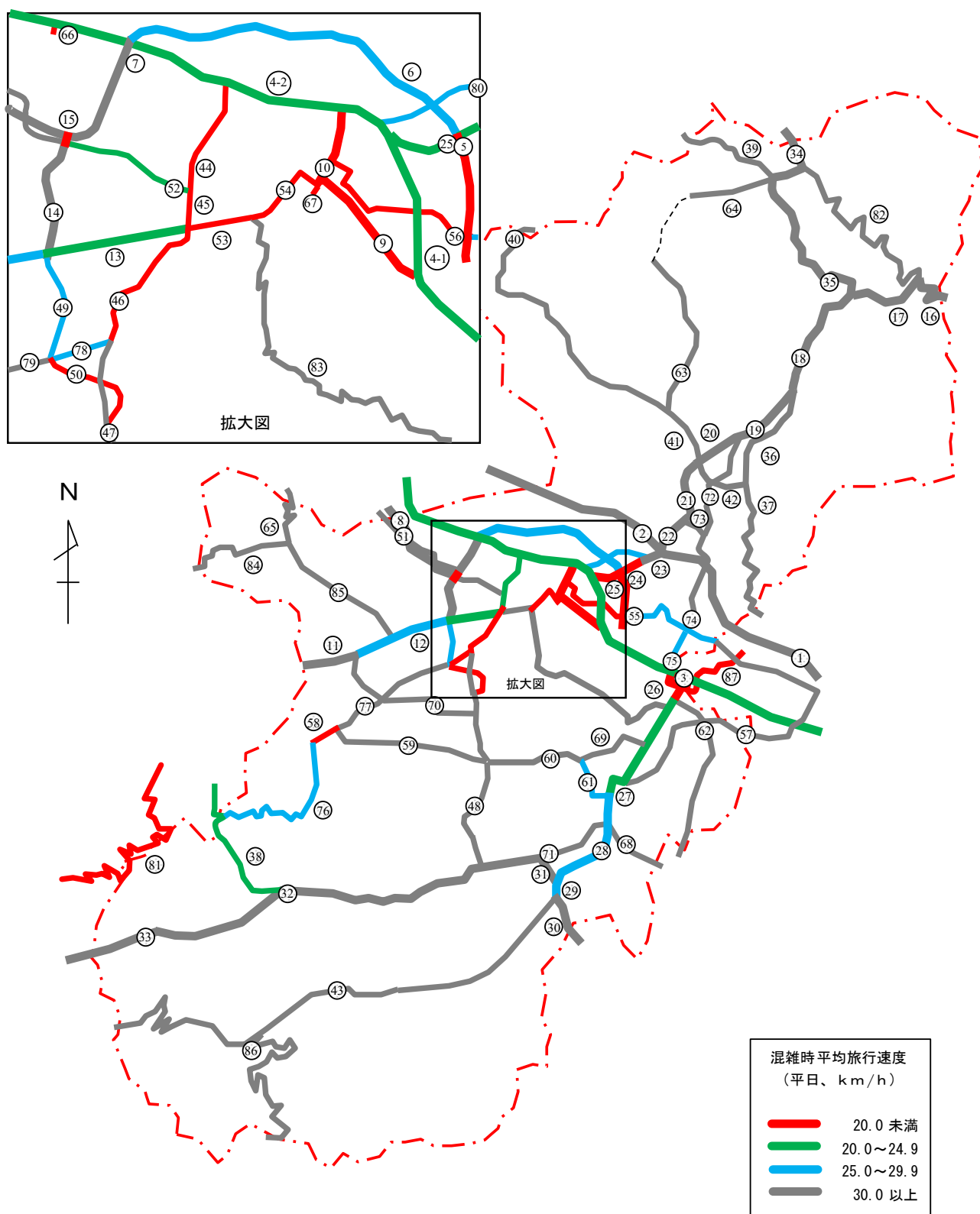
図6-1 混雑時平均旅行速度分布図(平均)
