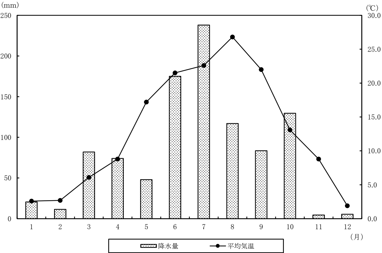
図8－2 気象概要(令和2年)
