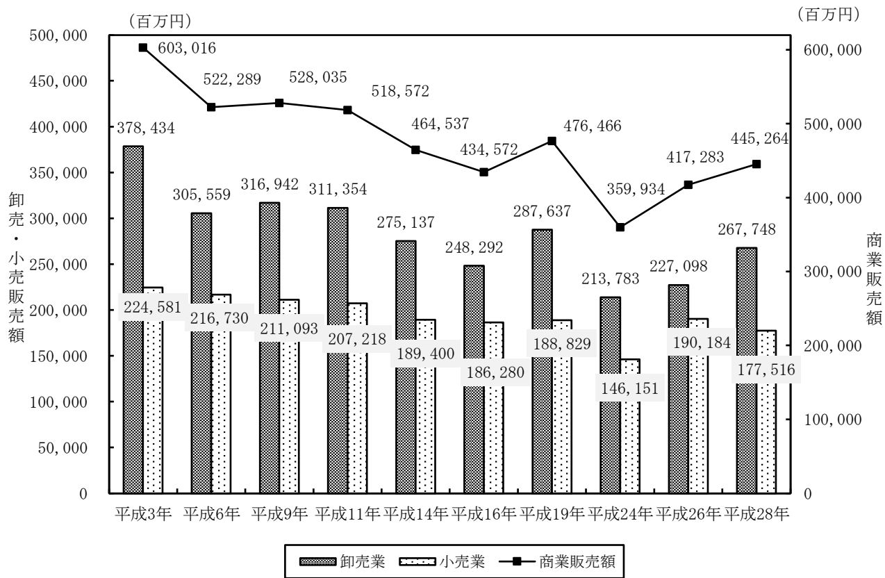
図2-11 業種別販売額の推移(デフレータ補正值)
