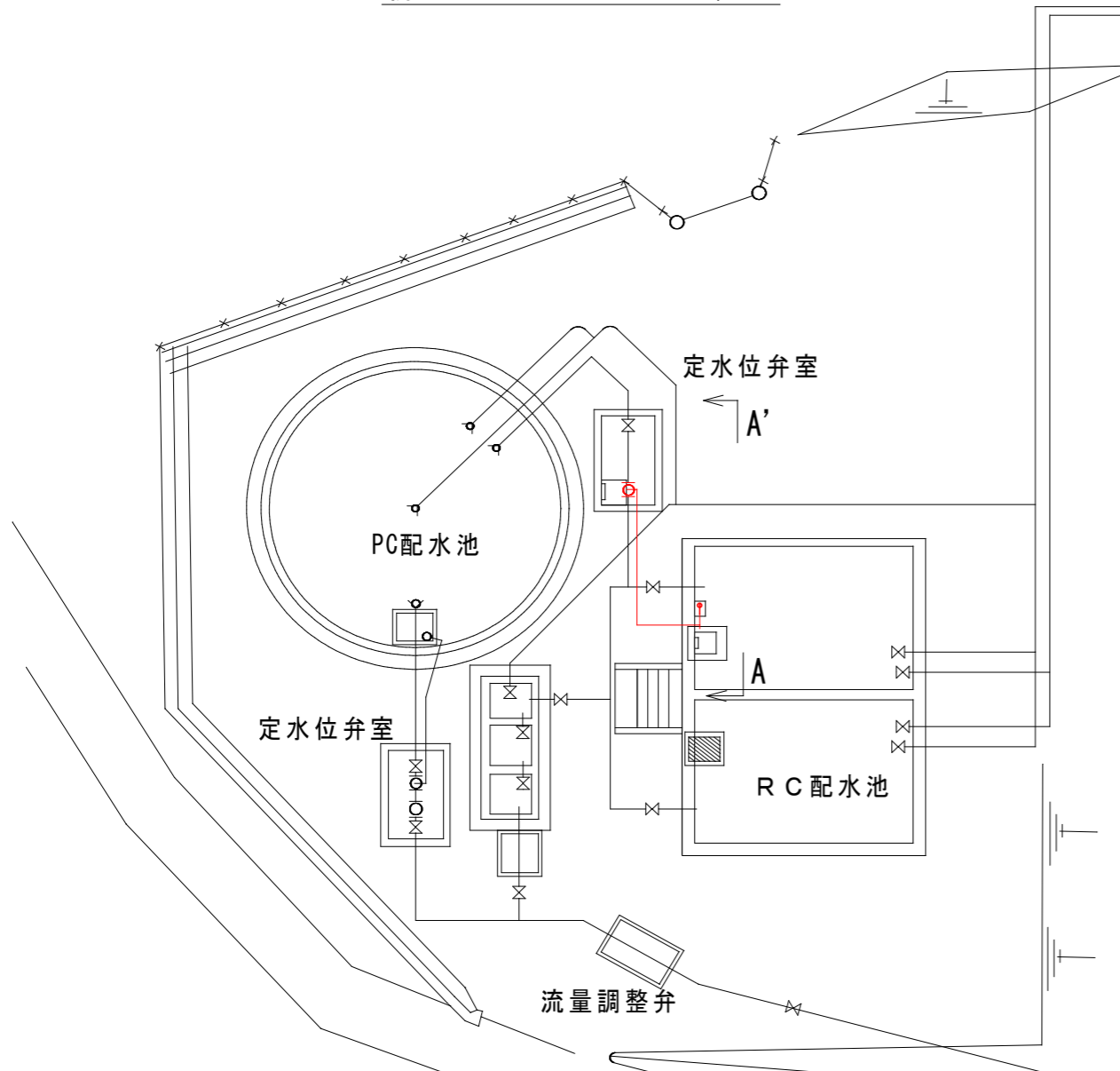
新屋配水池 平面図 S=1/160
