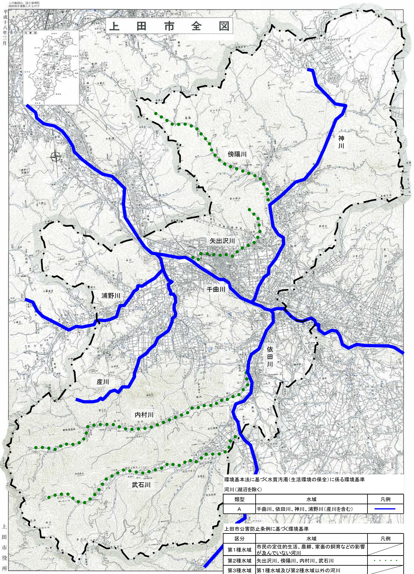
図1 水質汚濁に係る環境基準の水域類型指定図
