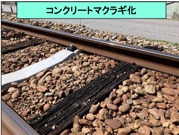
軌道道床硬質構造化
