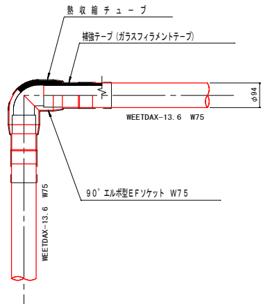
90° 曲管継手部詳細図 S=1:10
