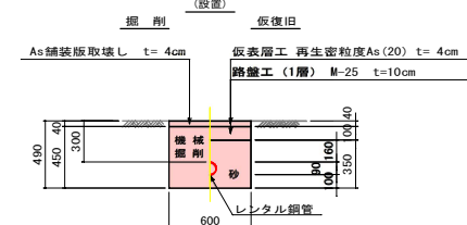
土工3-1：河川管理道As L=2.5m
