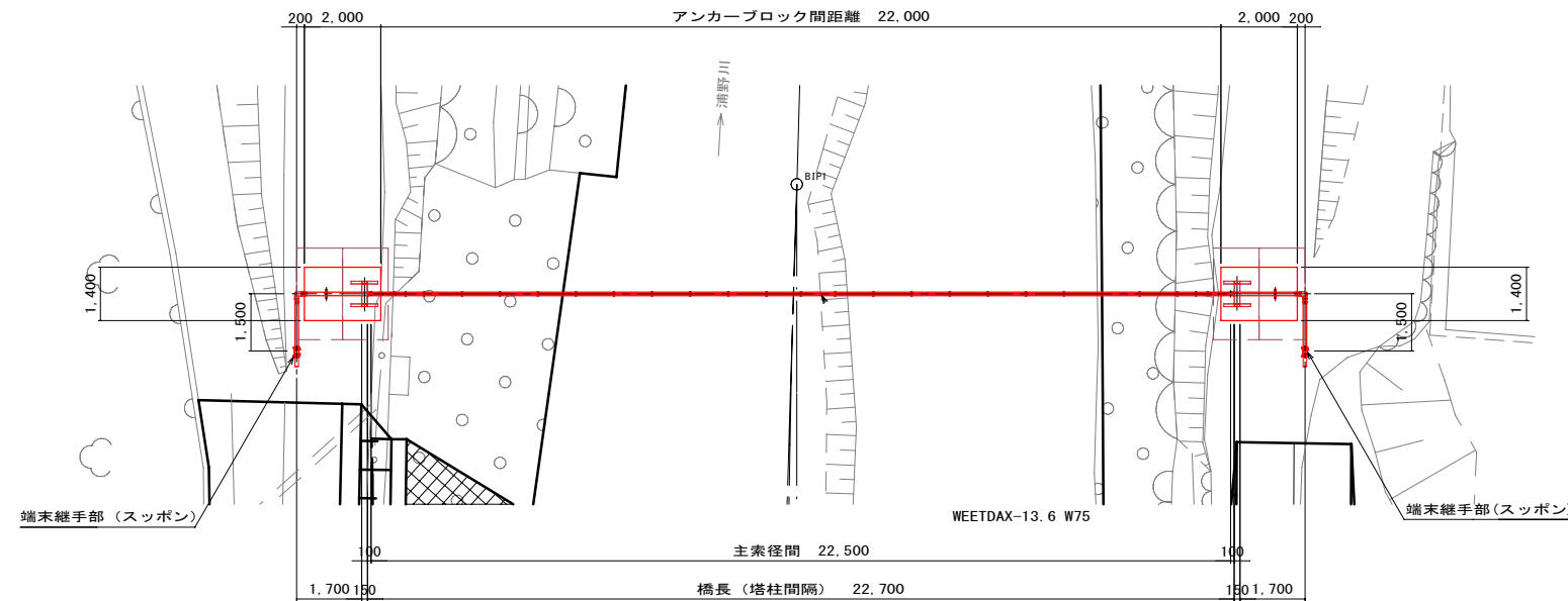
平面图 S=1:100
