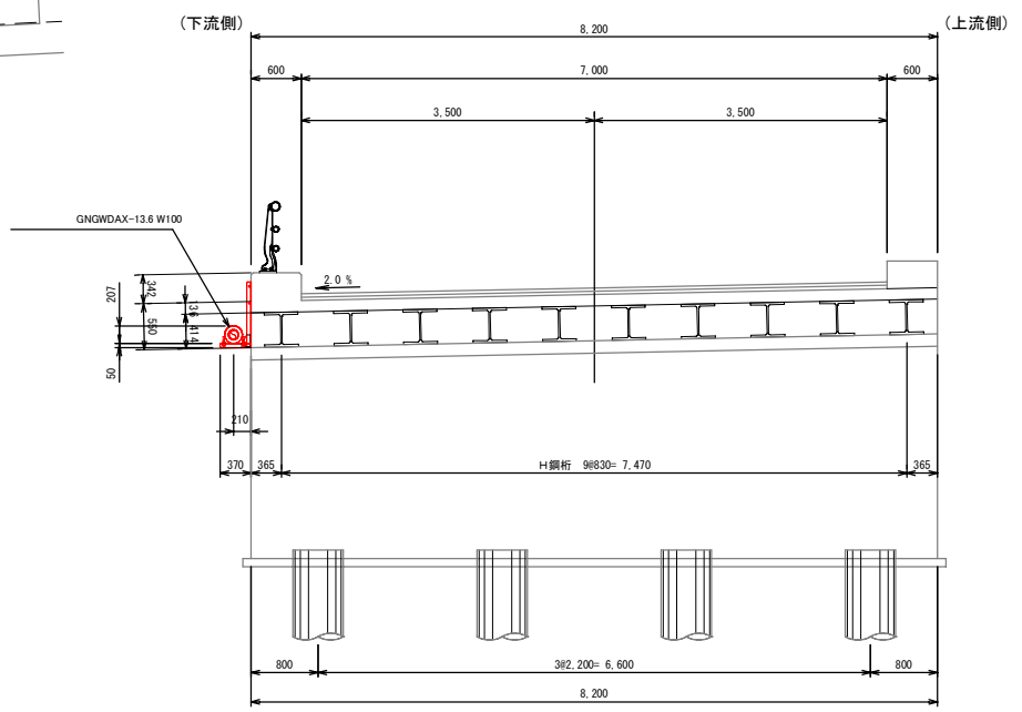
断面図 S=1:50
