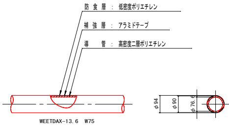
パイプ構造図 S=1:10
