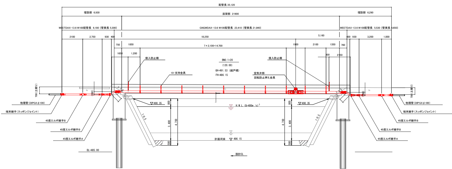
側面図 S=1:100
