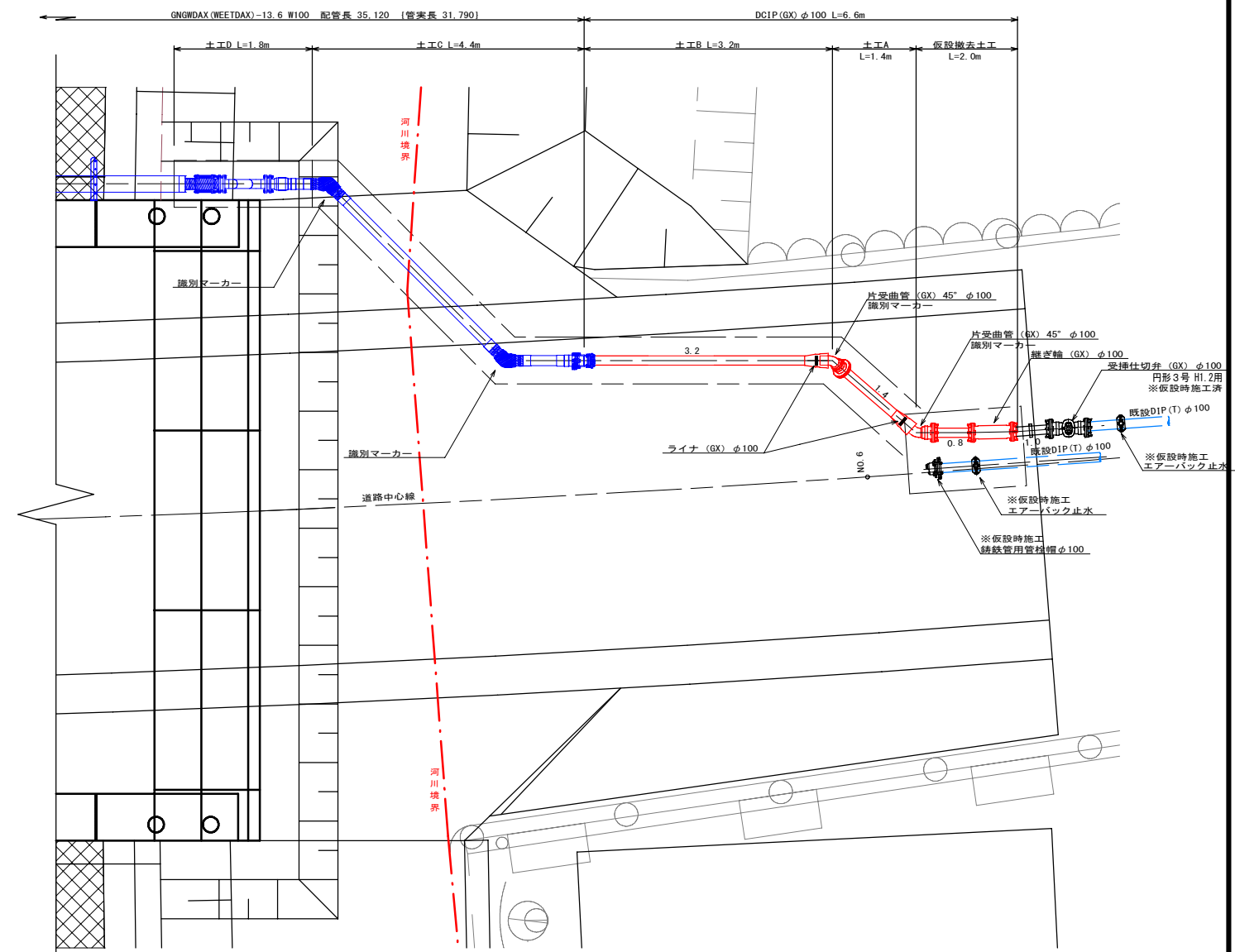
右岸側平面図
