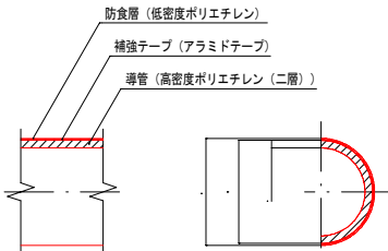
パイプ構造図
