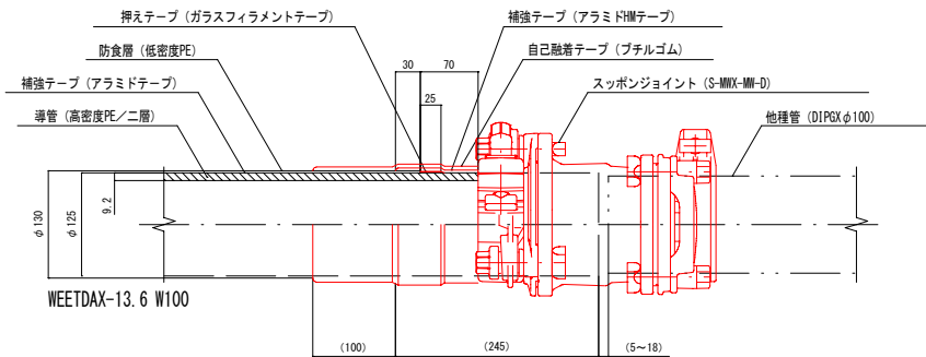
端末継手（スッポンジョイント）詳細図
