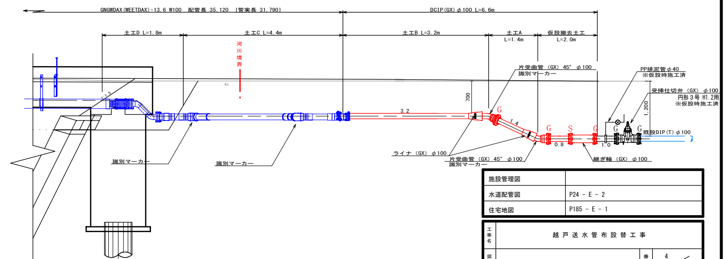
右岸側横断図
