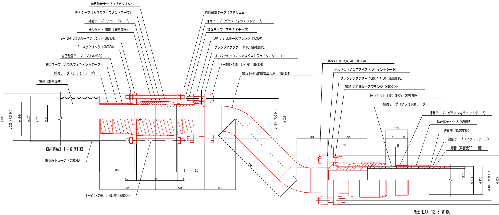
45度エルボ継手A（ロックリング・EF融着HM方式／JIS16Kフランジ）詳細図
