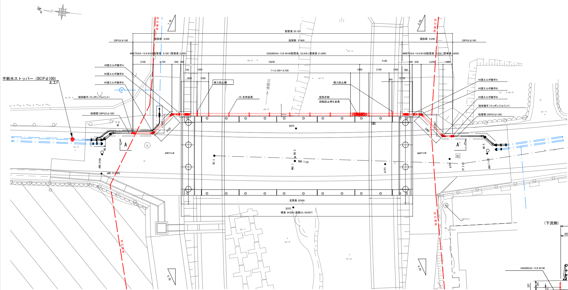
平面図 S=1:100
