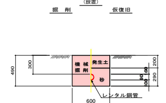
土工4-1：民地非鋪裝 L=16.6m
