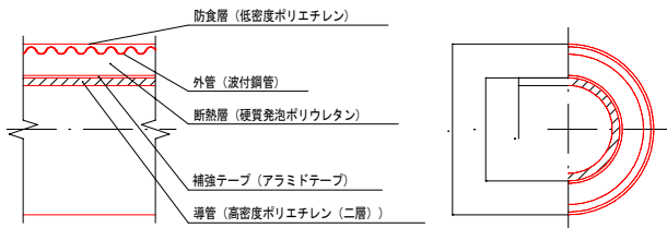
パイプ構造図
