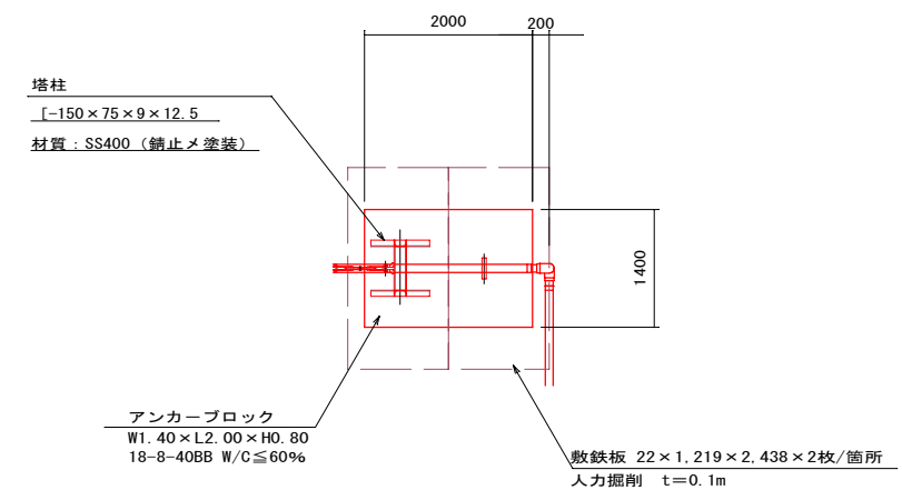
平面图 S=1:50
