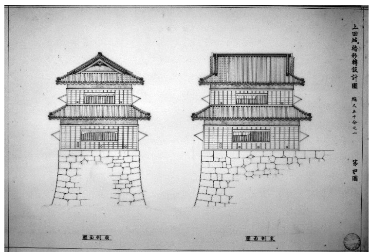
図 22 昭和 17 年(1942)「上田城櫓移転設計図 縮尺五十分之一 第四圖」 上田市教育委員会蔵
