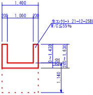
C-C断面
