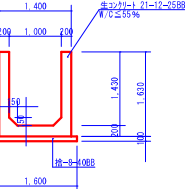
D-D断面
