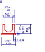
D-D断面
