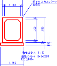
C-C断面
