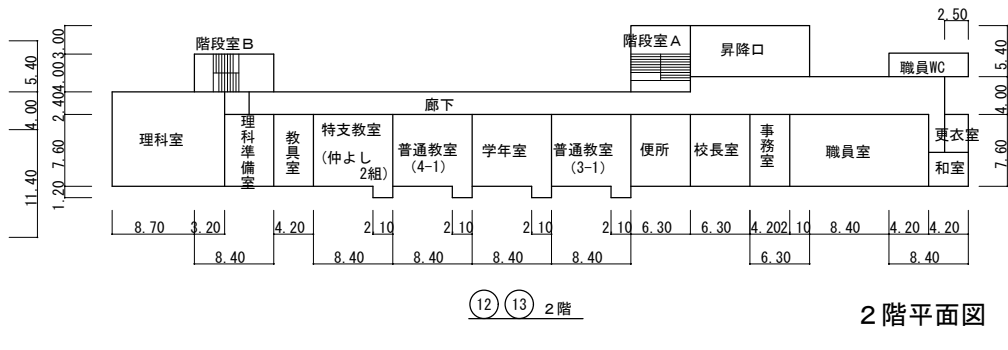
12 13 管理教室・特別教室棟 平面図 S=1/800
