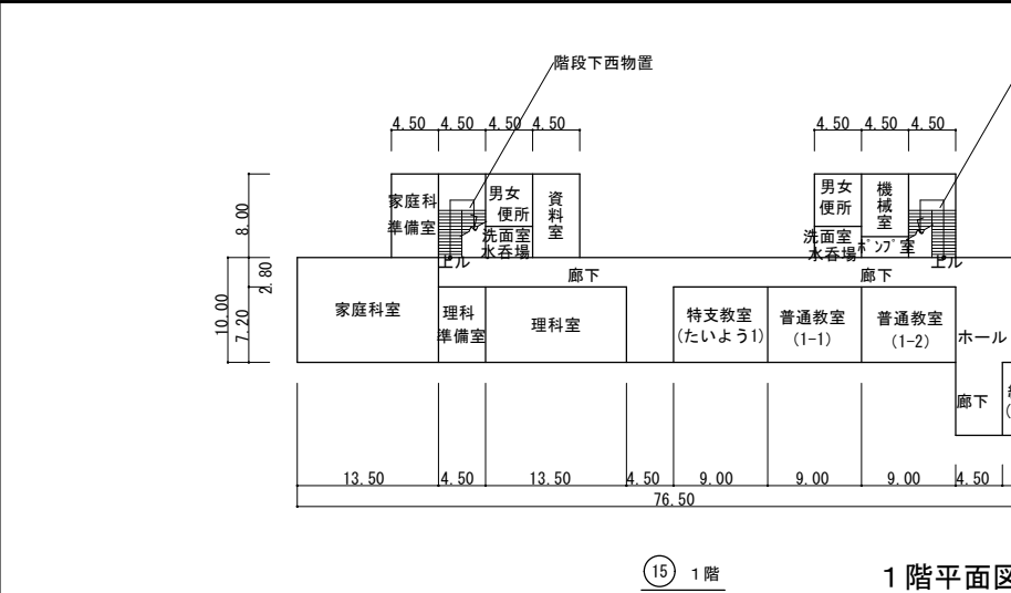
⑮ 1階平面図 ⑮ 普通・特別教室棟 平面図 S=1/800 (教室棟)
