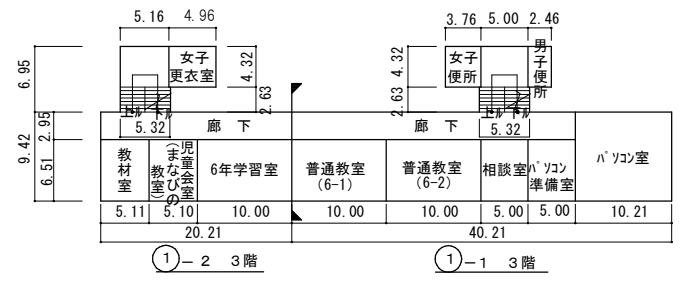
① 管理・教室棟 平面図 S=1/800 (第一校舎)
