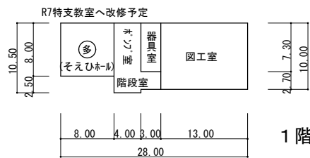
22 特別教室棟 平面図 S=1/800
