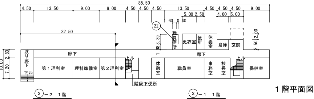
② 管理・特別教室棟 平面図 S=1/800 (中校舎)
