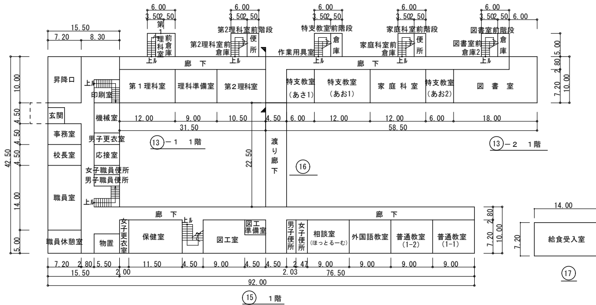
⑬⑮ 教室棟、管理棟、特別・普通教室棟 平面図 S=1/800
