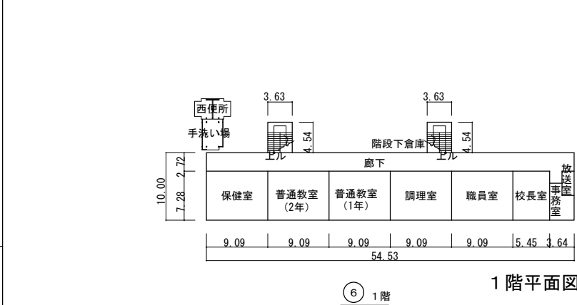
6 普通・特別教室棟 平面図 S=1/800 (南校舎)
