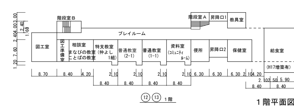
12 13 管理教室・特別教室棟 平面図 S=1/800
