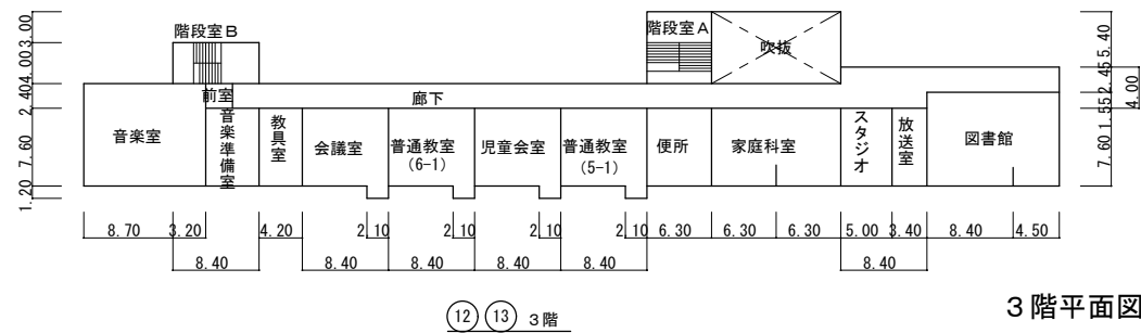
⑫⑬ 管理教室・特別教室棟 平面図 S=1/800
