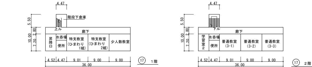
1 階平面図 2 階平面図 普通教室棟 平面図 S=1/800 (東校舎)
