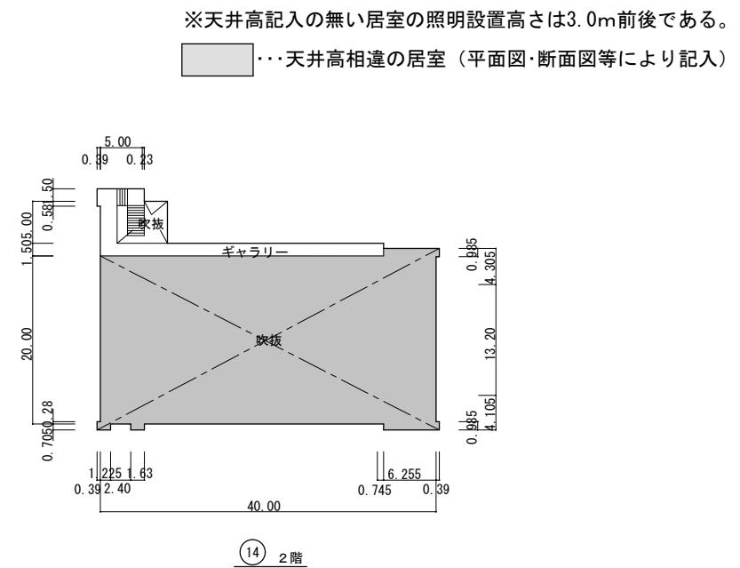
⑭ 屋内運動場 平面図 S=1/800
