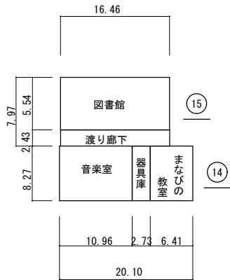
15 図書館棟 平面図 S=1/800
