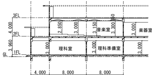
35 特別教室棟 断面図 S=1/500
