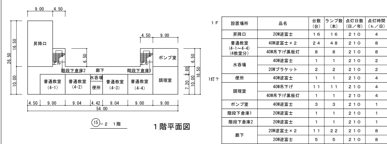
普通教室棟 平面図 S=1/800 (北校舎)
