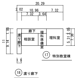
17 18 特別教室棟 平面図 S=1/800
