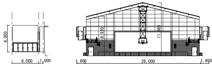
18 屋内運動場 展開図 S=1/500
