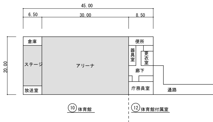
10 12 屋内運動場 平面図 S=1/800
