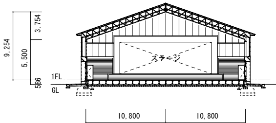
13 屋内運動場 断面図 S=1/500
