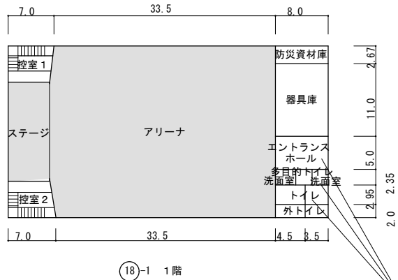
18 屋内運動場 平面図 S=1/800
