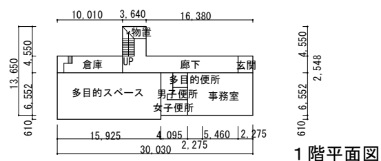
清明児童クラブ 平面図 S=1/800
