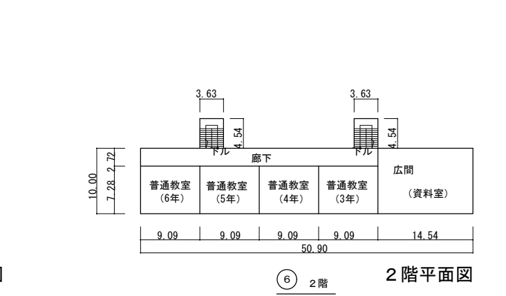
6 普通・特別教室棟 平面図 S=1/800 (南校舎)
