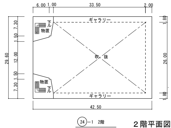
②④ 屋内運動場 平面図 S=1/800
