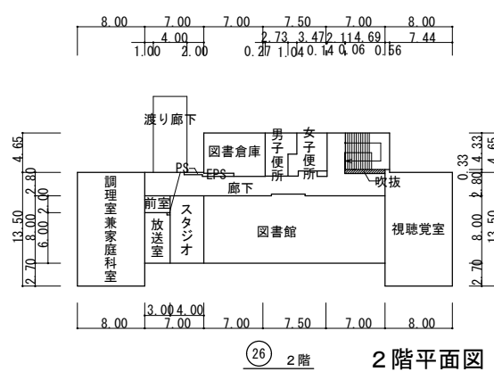
26 管理棟 平面図 S=1/800 (管理棟)
