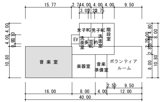
35 2階
