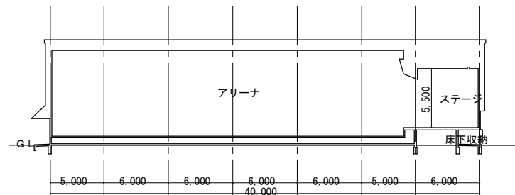
⑭ 屋内運動場 断面図 S=1/500
