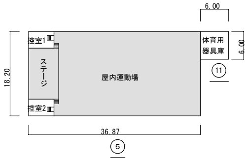
5 11 屋内運動場 平面図 S=1/800
