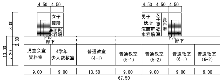
15 3階平面図
