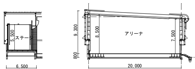
10 12 屋内運動場 矩計図 S=1/500
