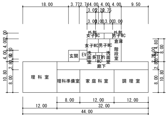
35 1階
