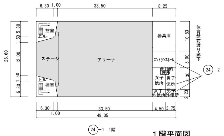
②④ 屋内運動場 平面図 S=1/800
