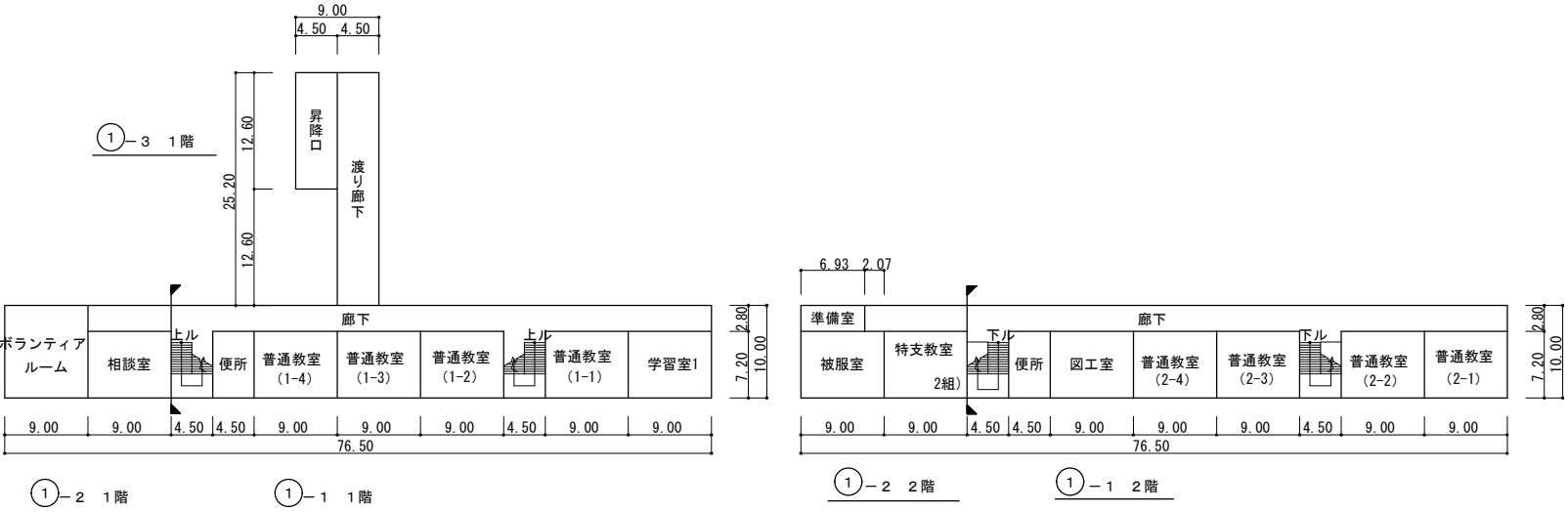
1階平面図
