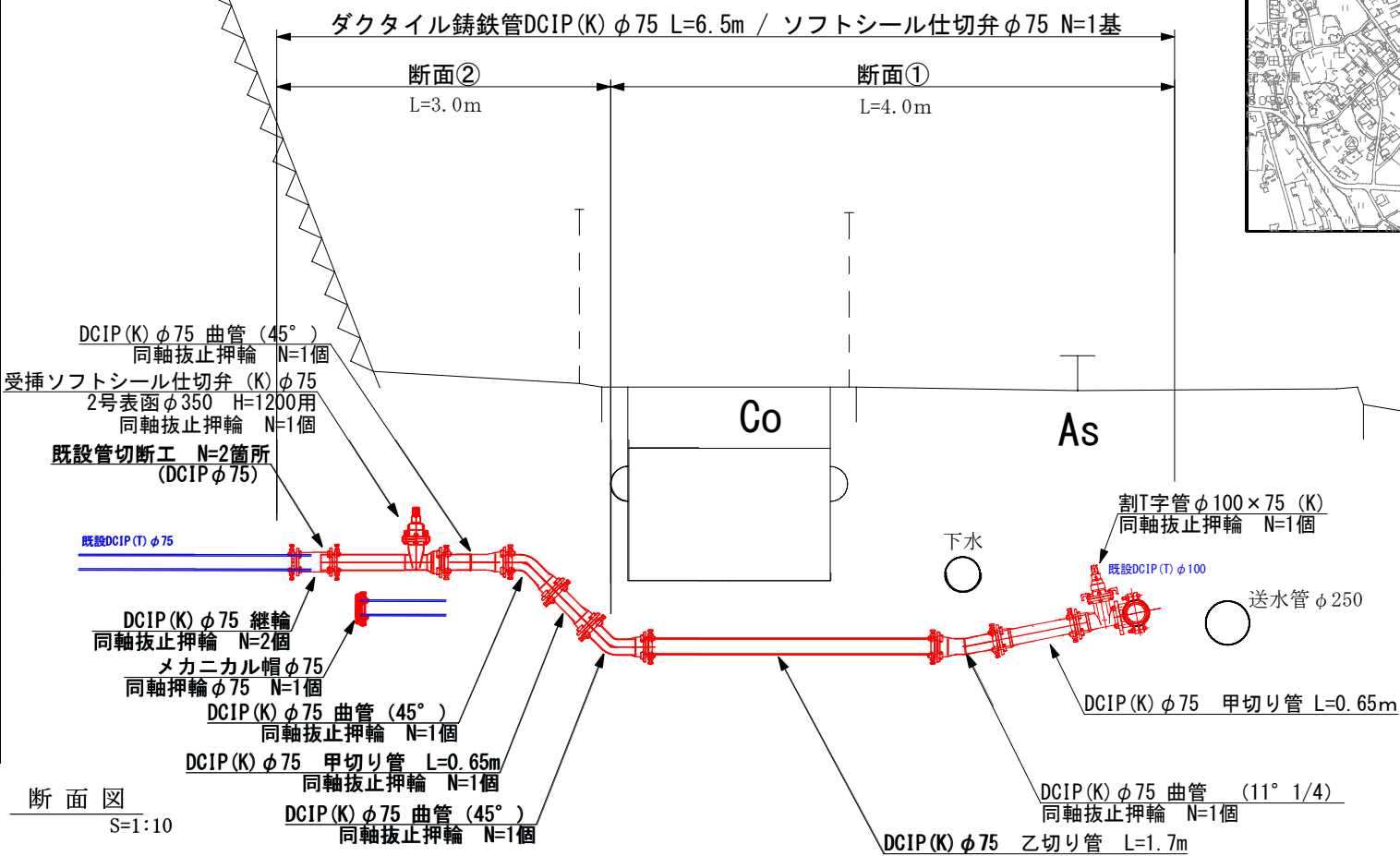
断面② L=3.0m
