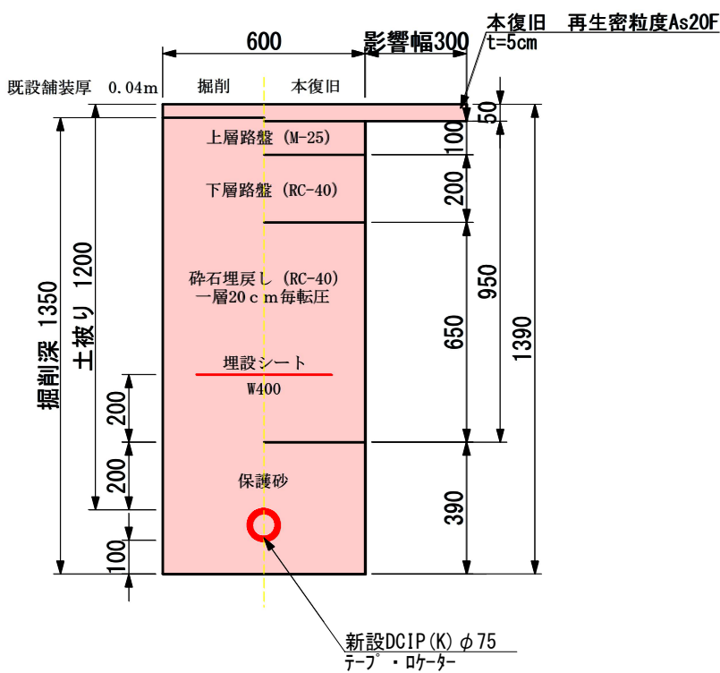
断面② L=3.0m
