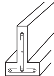
鉄筋コンクリート 布基礎の代表例
