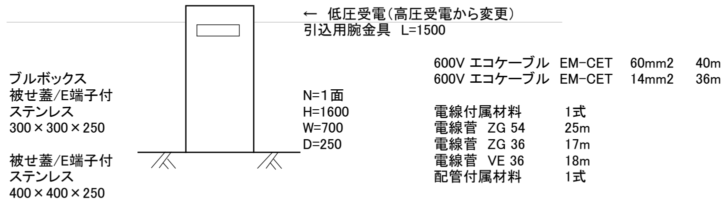
引込開閉器盤 (参考)
