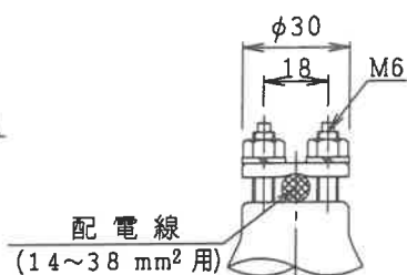
端子部詳細図
