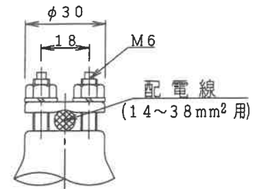
端子部詳細図
