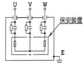
内部結線図
