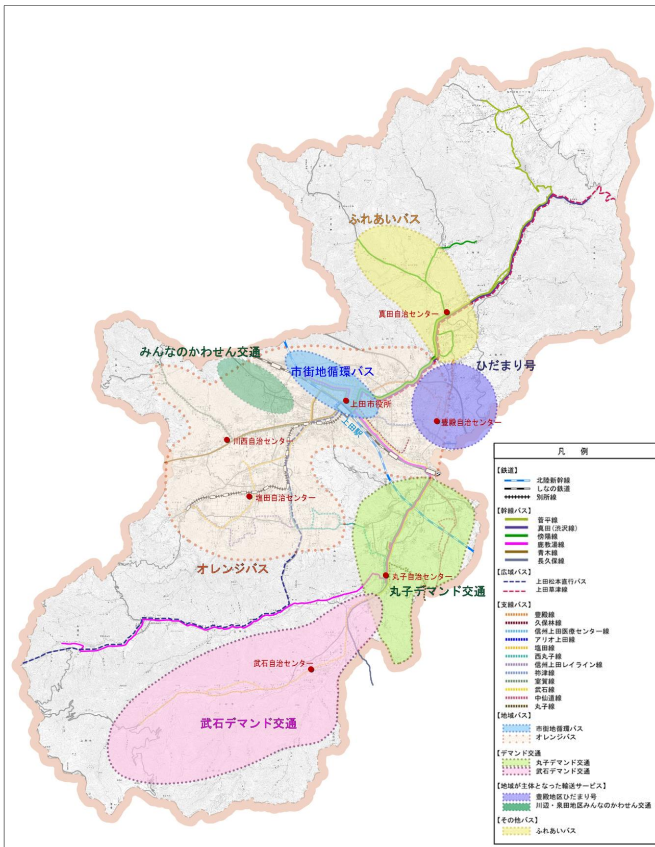
図 3-1 市内における地域公共交通の体系
