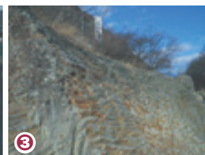
流紋岩の柱状節理
