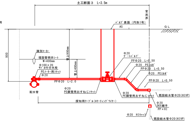
給水 3 No. 2+27付近 左
