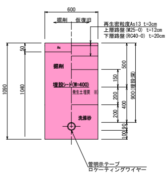
土工断面 2
