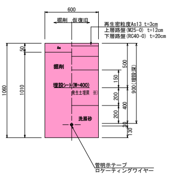
(給水) 土工断面 3
