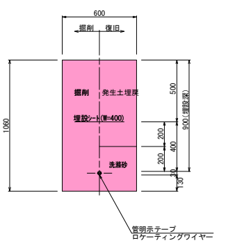
(給水) 土工断面 4
