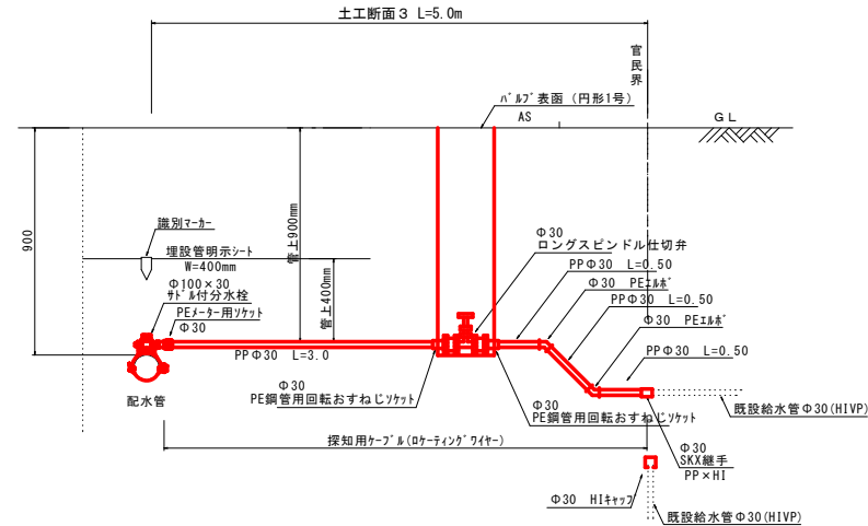
給水 5 No. 2+27付近 左
