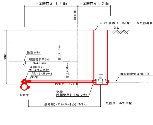
給水 5 No. 2+27付近 左
