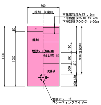
土工断面 1
