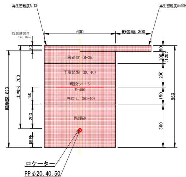
土工断面1 L=67.5m (市道 As) φ20, 40, 50
