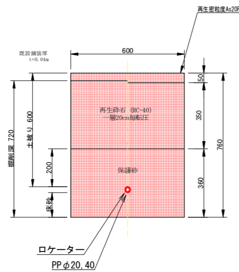
土工断面2 L=14.5m (民地 As) φ20, 40
