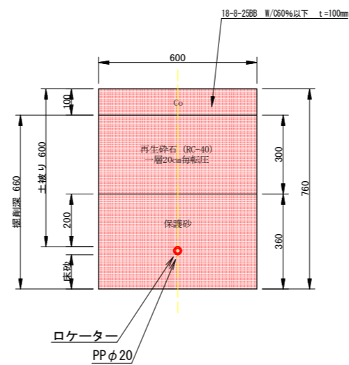
土工断面3 L=6.0m (民地 Co) φ20
