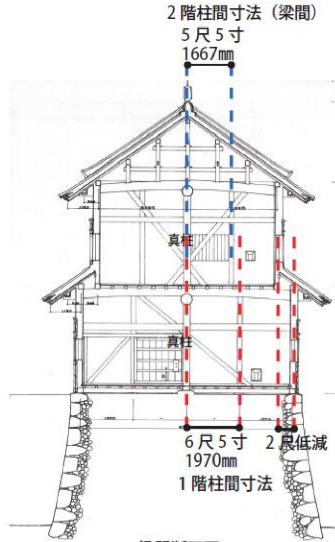
梁間断面図
