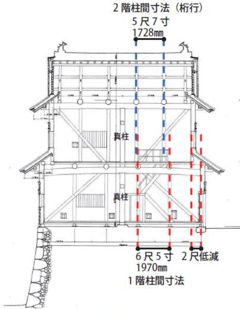
桁行断面図
