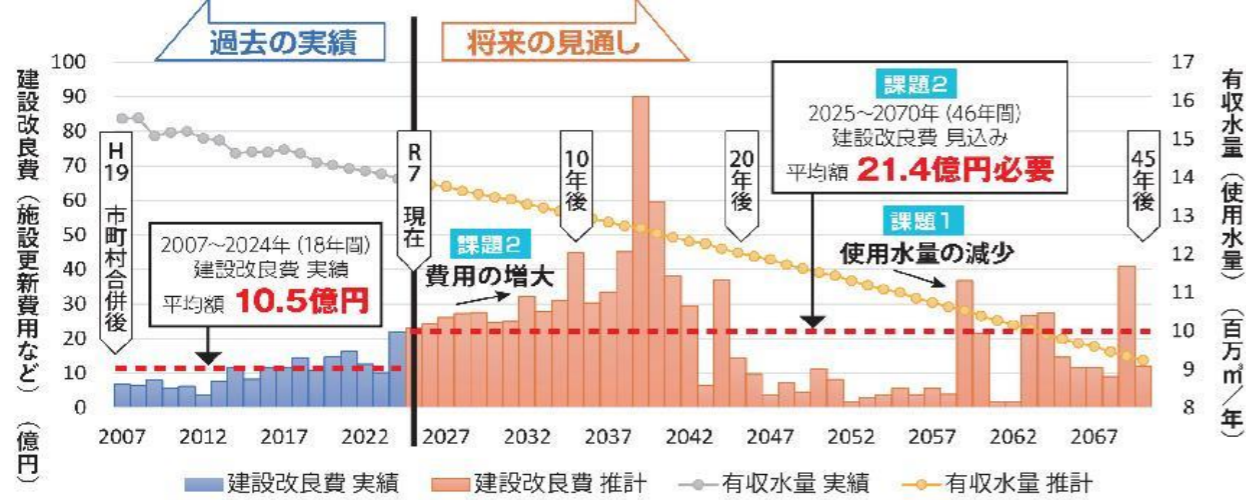
■市営水道の施設更新費用・使用水量の状況
