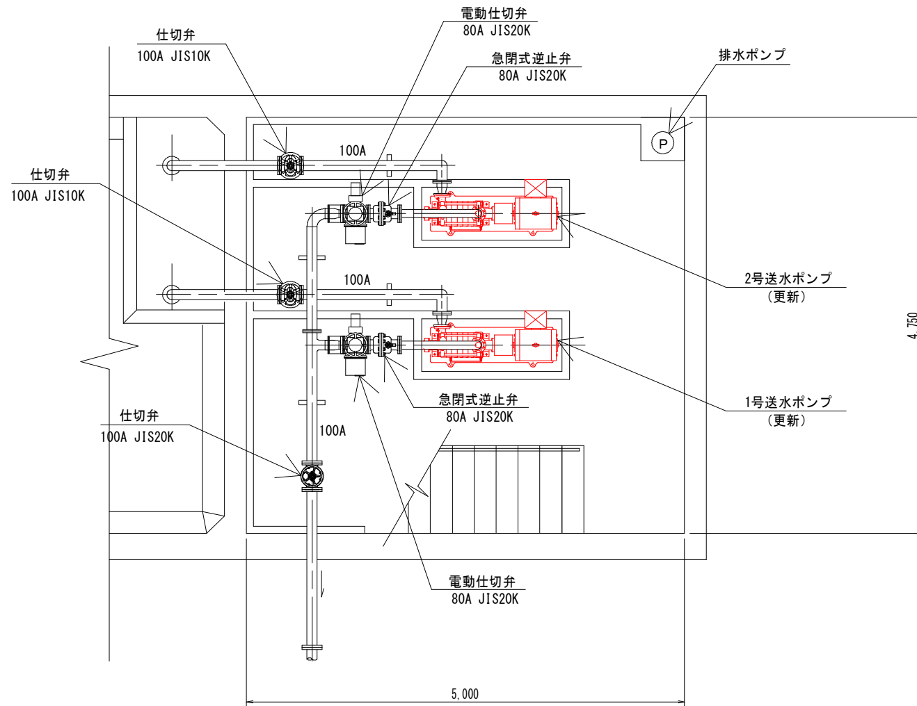
機器据付配管平面図 S=1/60
