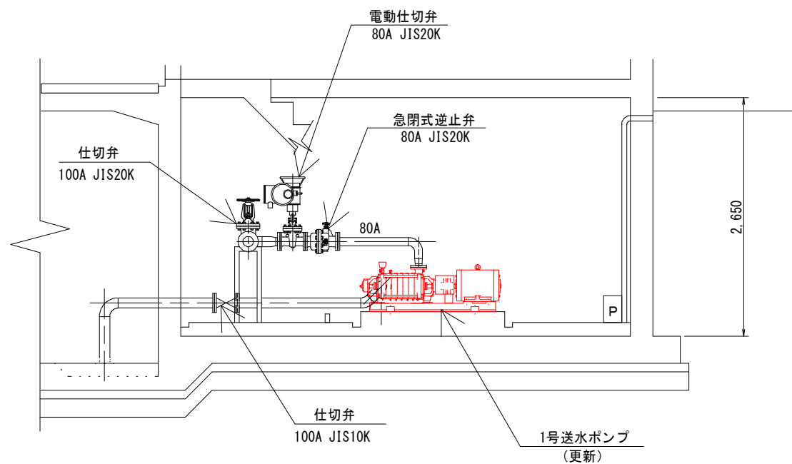
機器据付配管断面図 S=1/60
