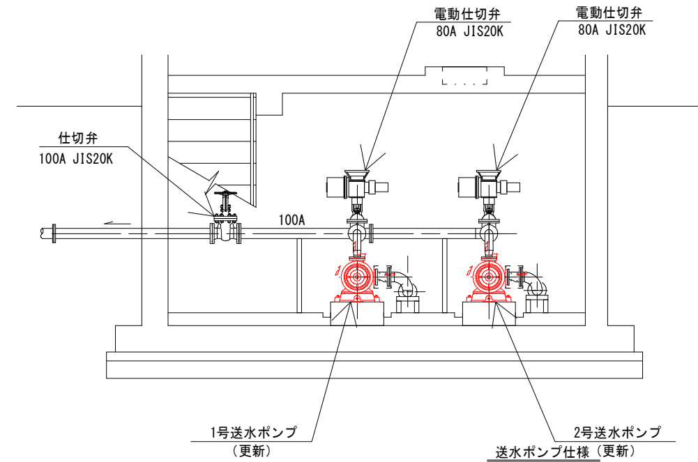
機器据付配管断面図 S=1/60
