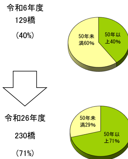
アセットマネジメント橋梁323橋の 高齢化の推移（令和6年度→20年後）
