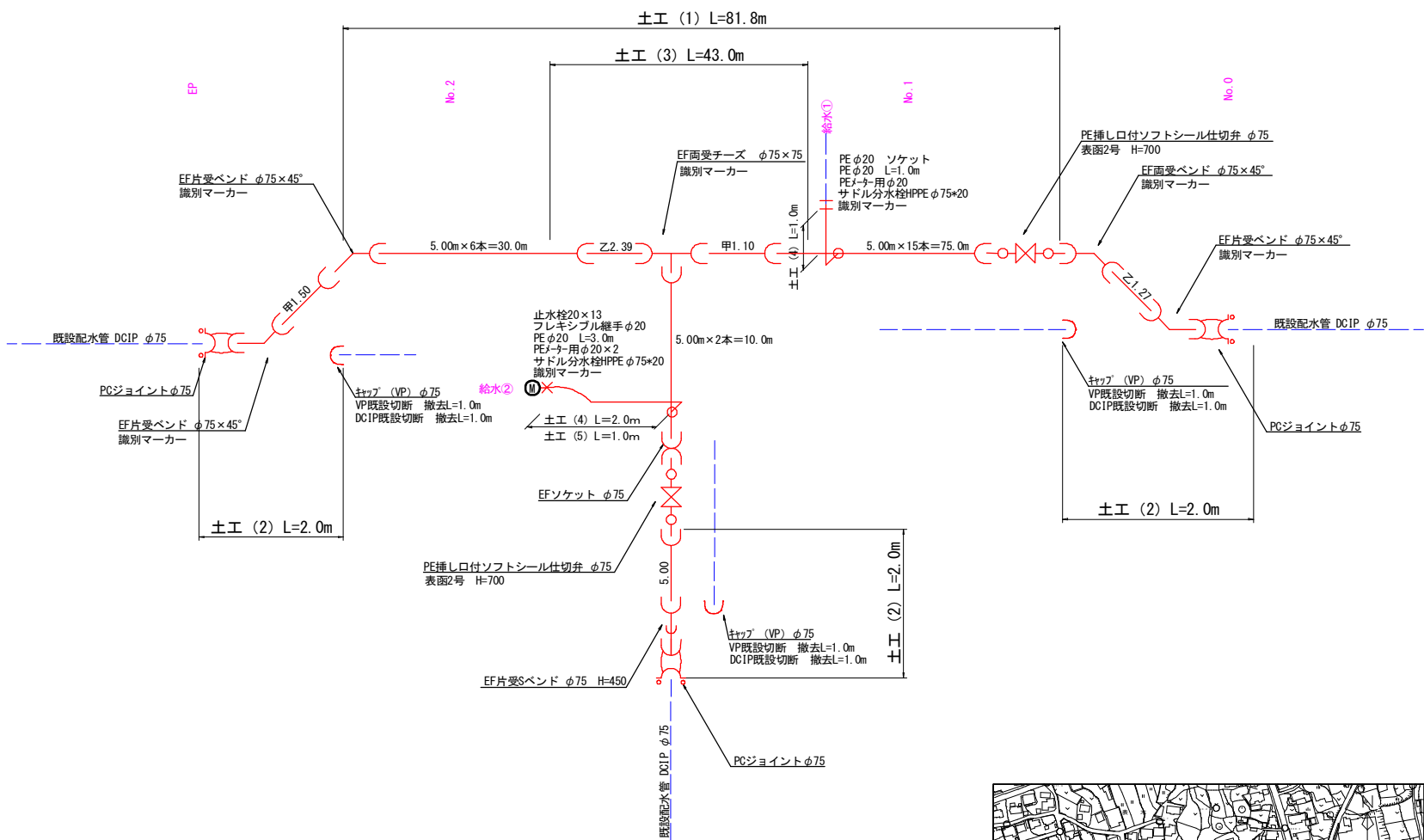
配管詳細図 S=FREE
