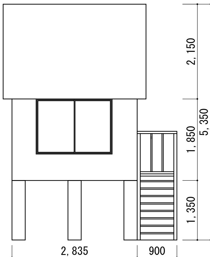
東立面図
