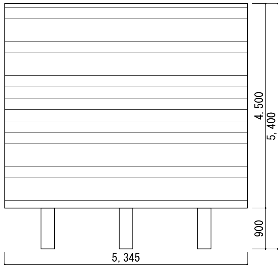
東立面図
