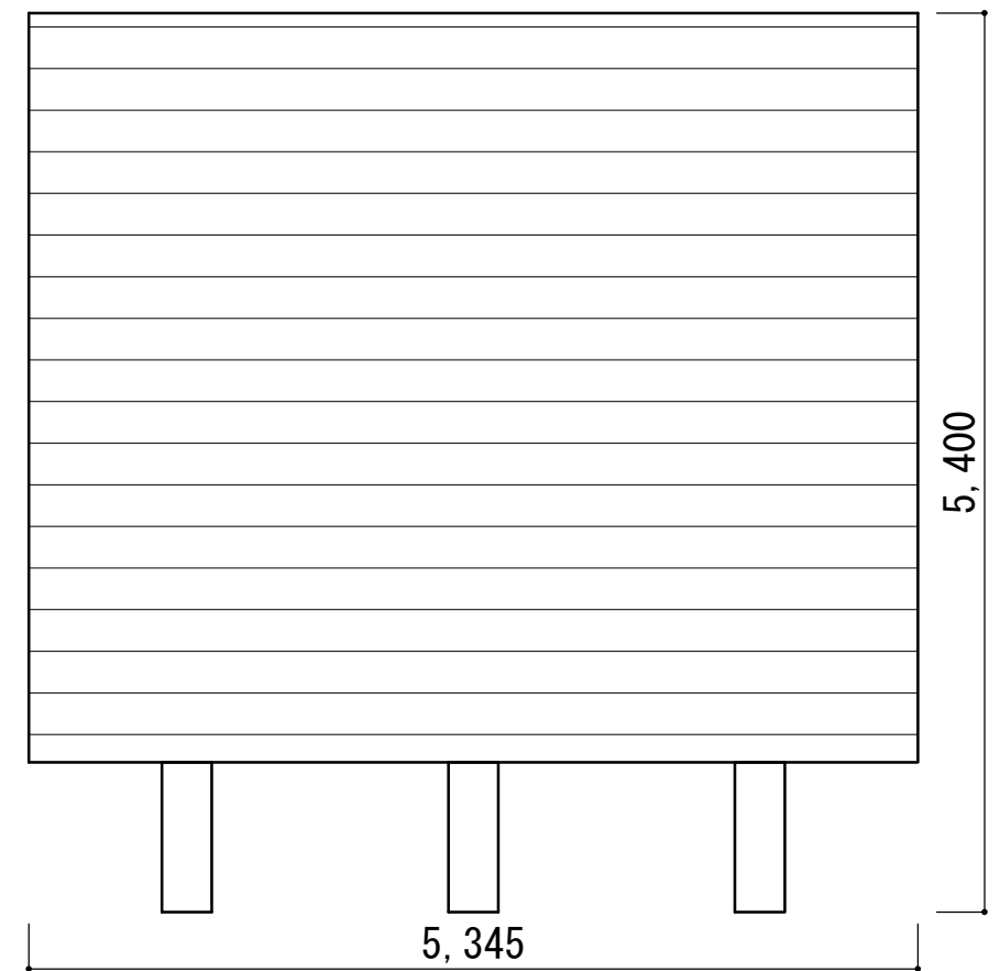
西立面図
