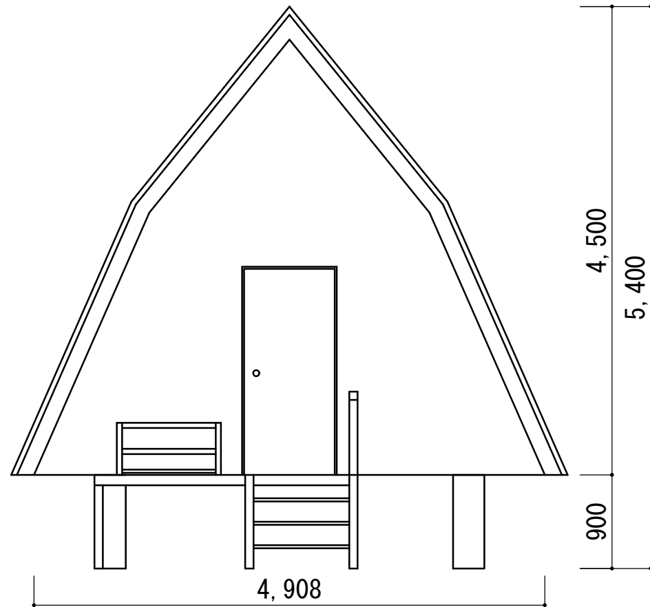
北立面図
