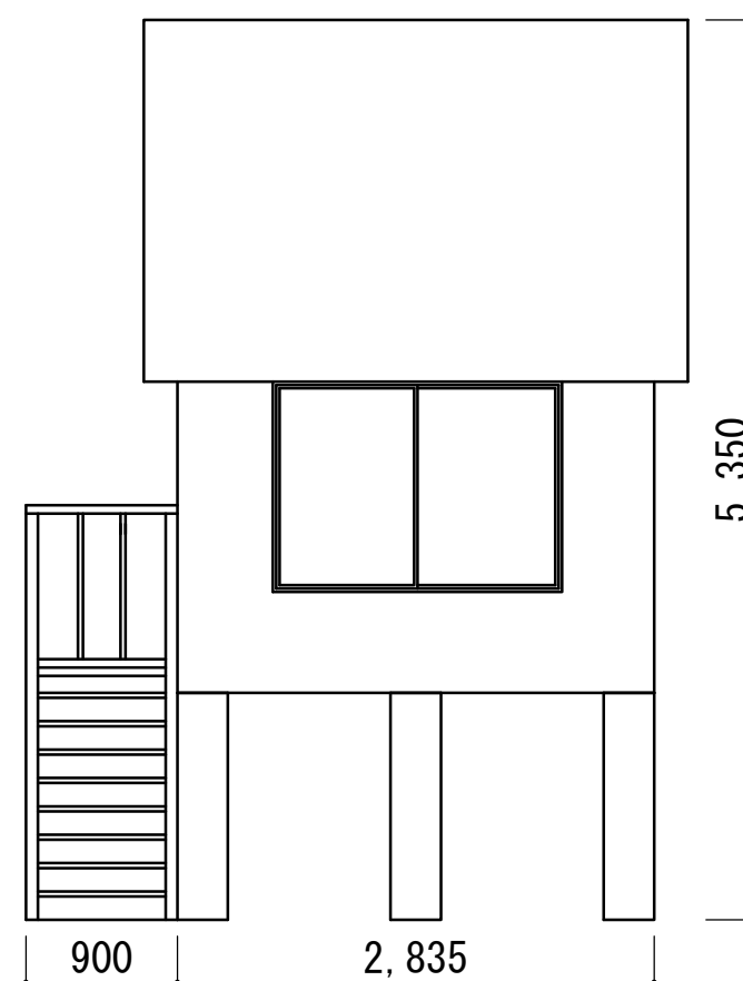
西立面図
