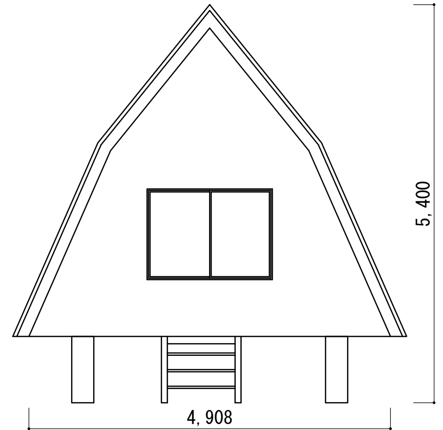
南立面図
