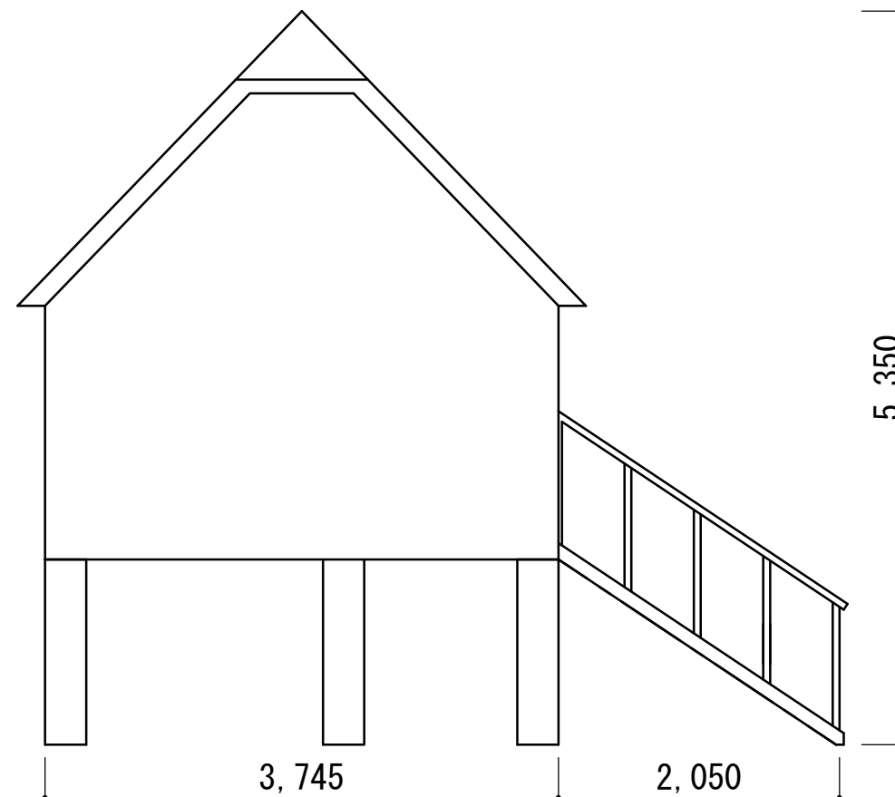
南立面図
