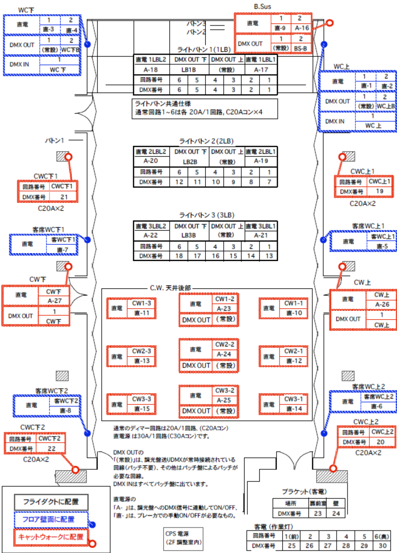
ASPINA 文化ホール(上田市丸子文化会館)小ホール照明回路図
