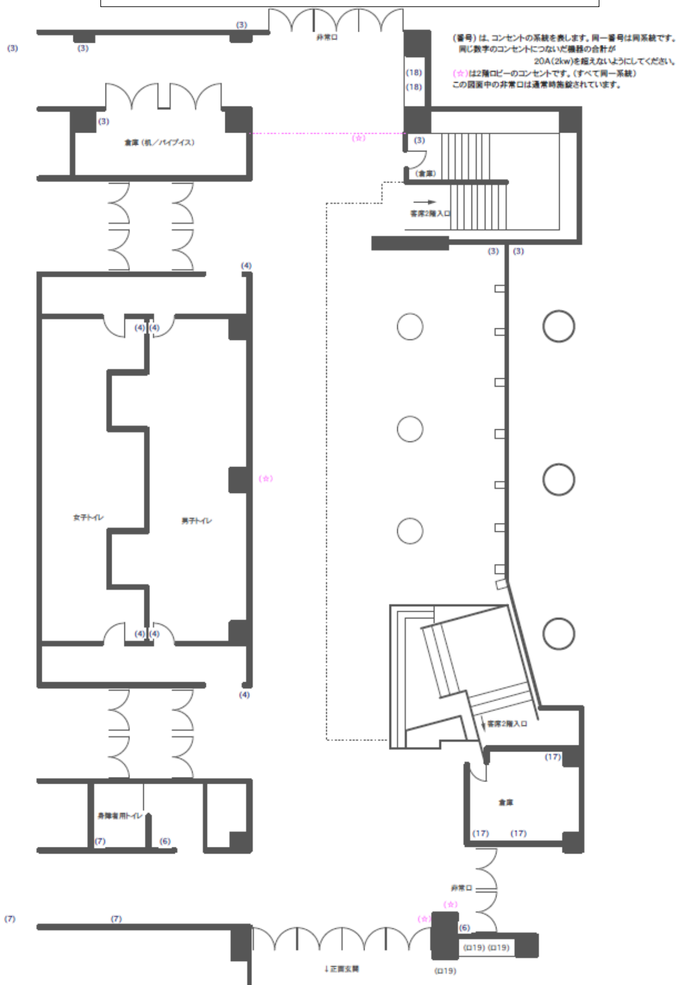
ASPINA 文化ホール(上田市丸子文化会館)大ホールホワイエ平面図
