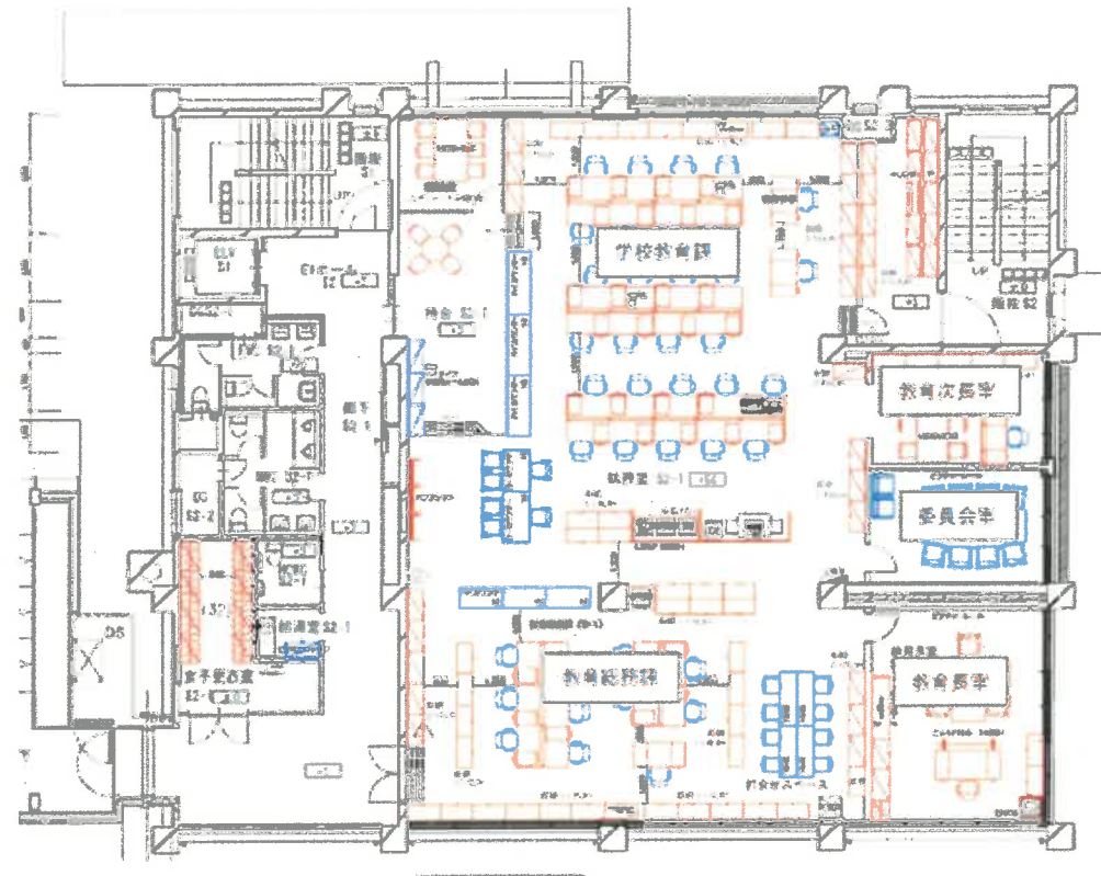
2階平面図
